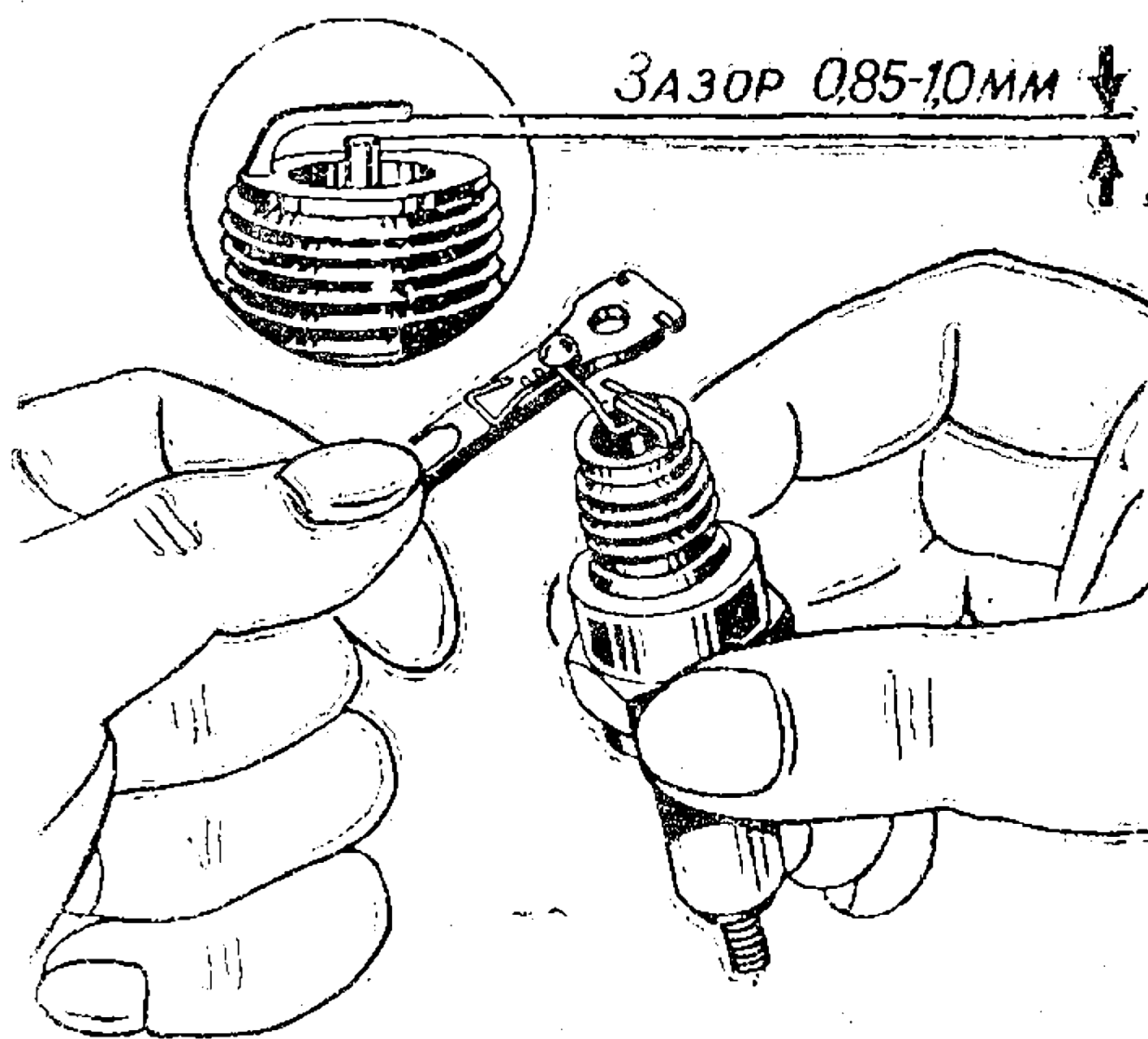
Рис. 58. Проверка зазора между электродами свечи
