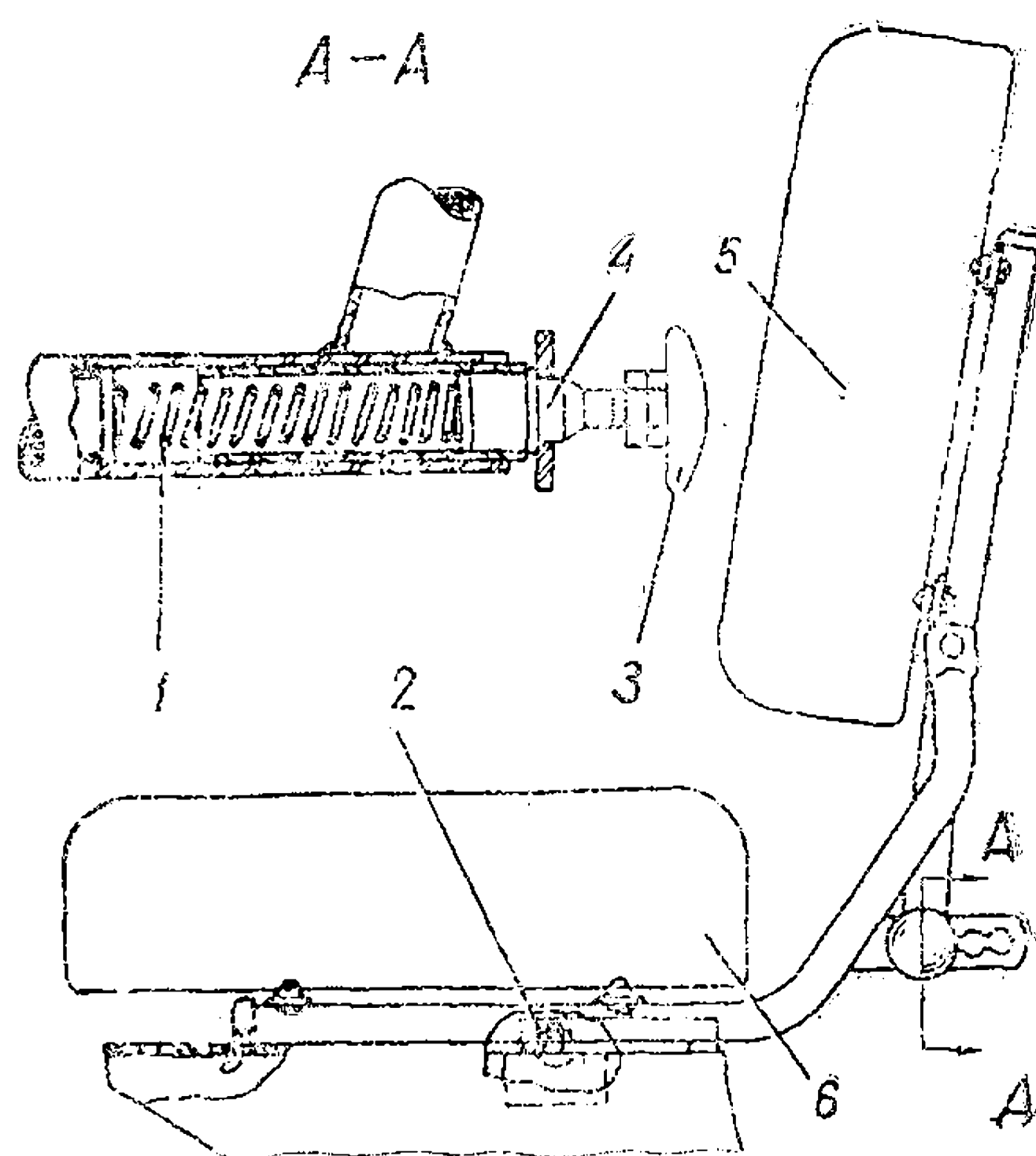
Рис. 74. Сиденье:
