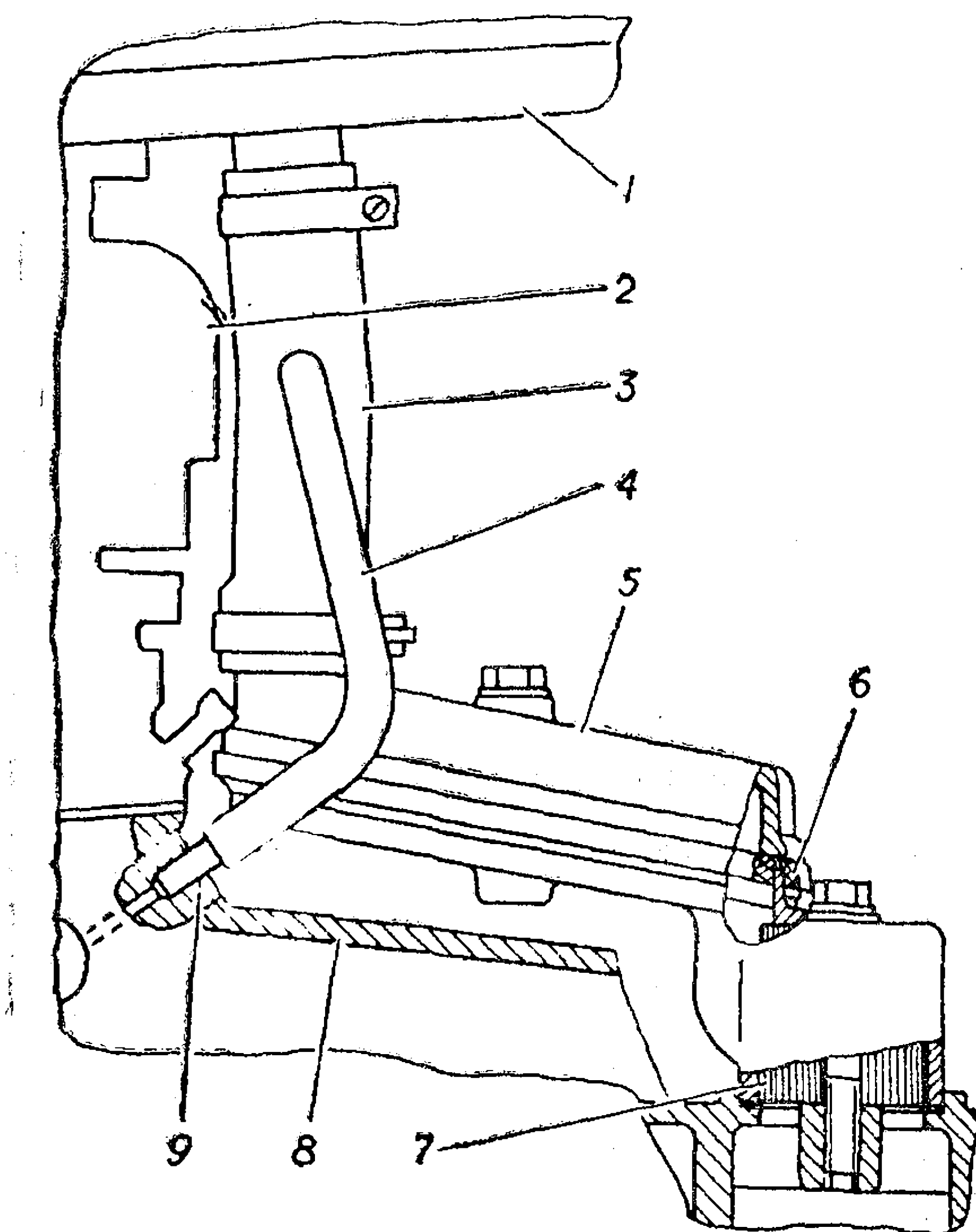
Рис. 13. Схема закрытой системы вентиляции картера:
