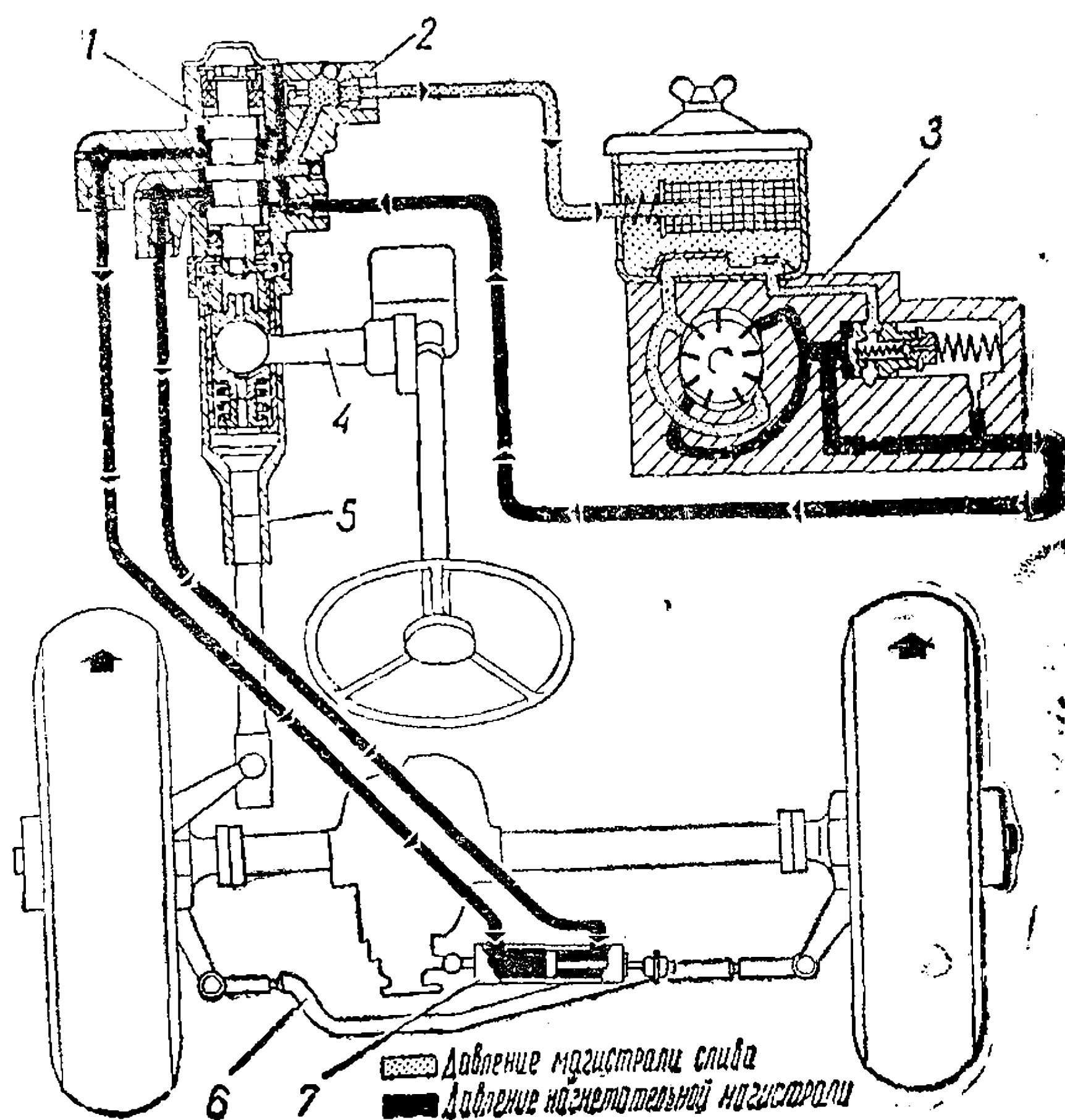
Рис. 47. Схема работы гидросилителя рулевого привода. Движение по прямой:
