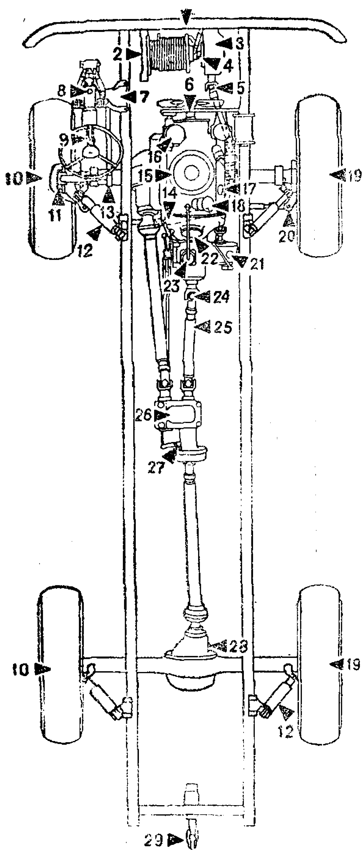
Рис. 101. Места смазки автомобиля
