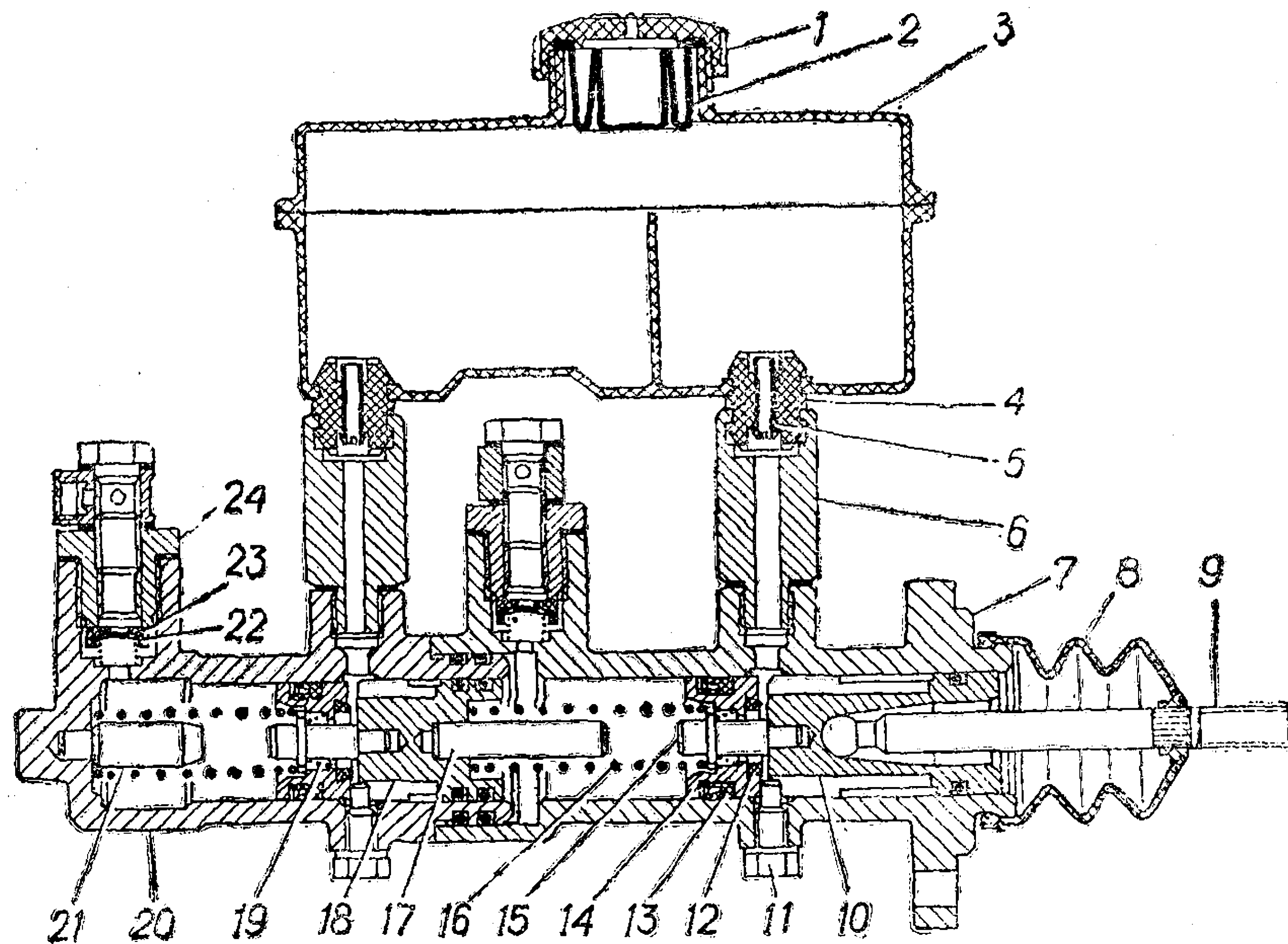
Рис. 51. Главный цилиндр:
