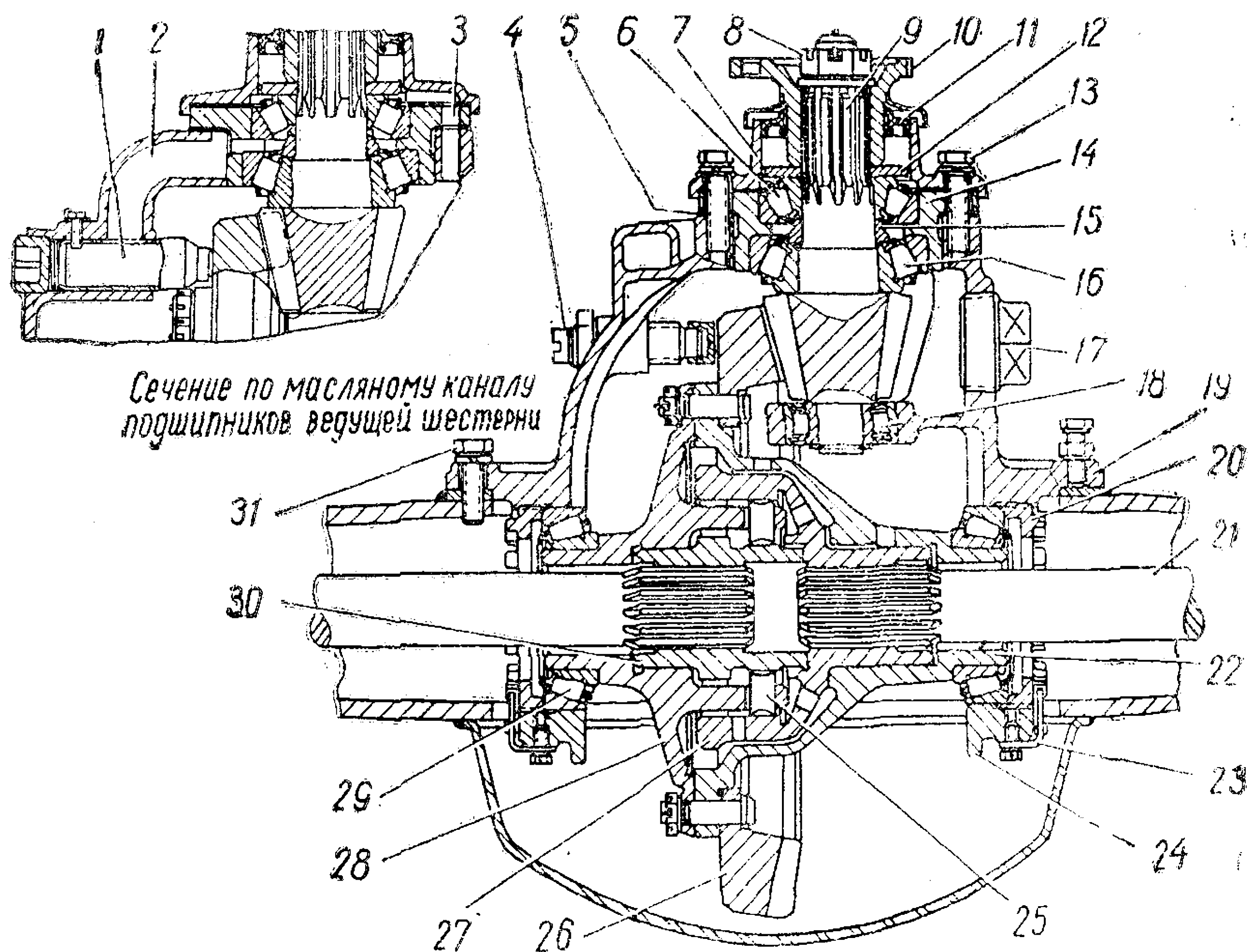
Рис. 30. Главная передача:
