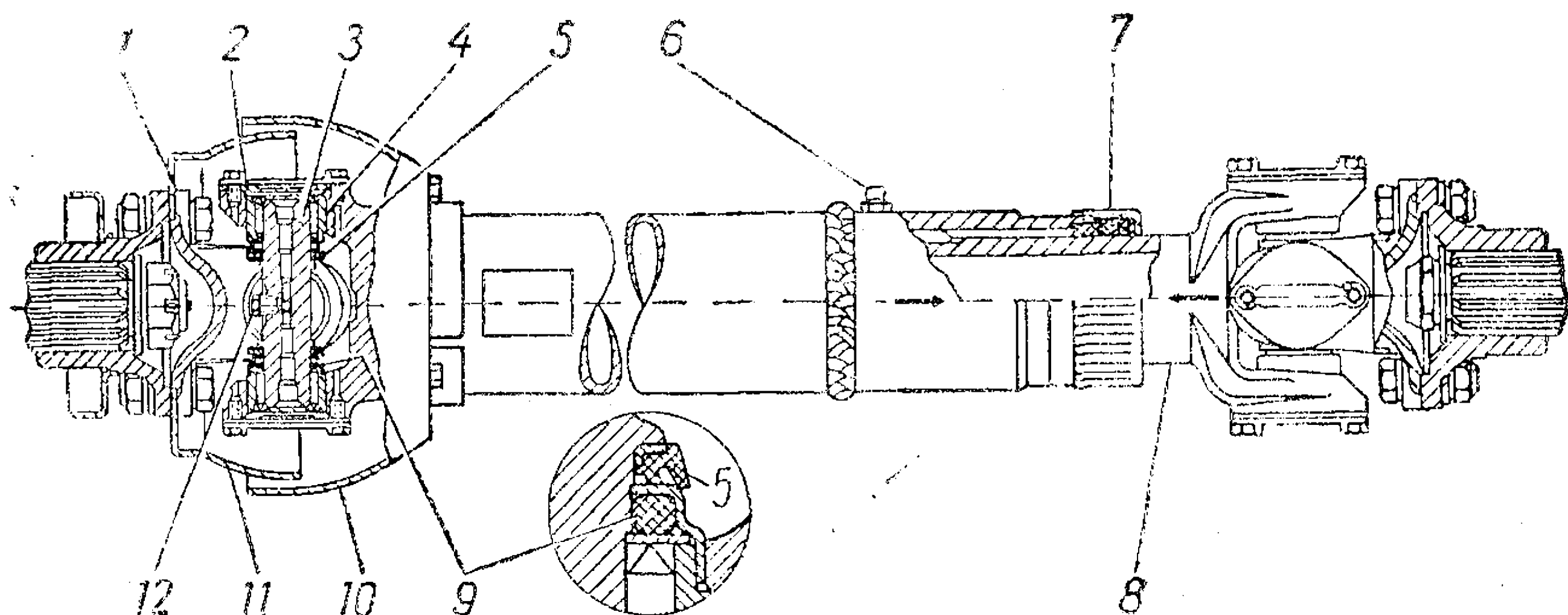
Рис. 27. Карданный вал:
