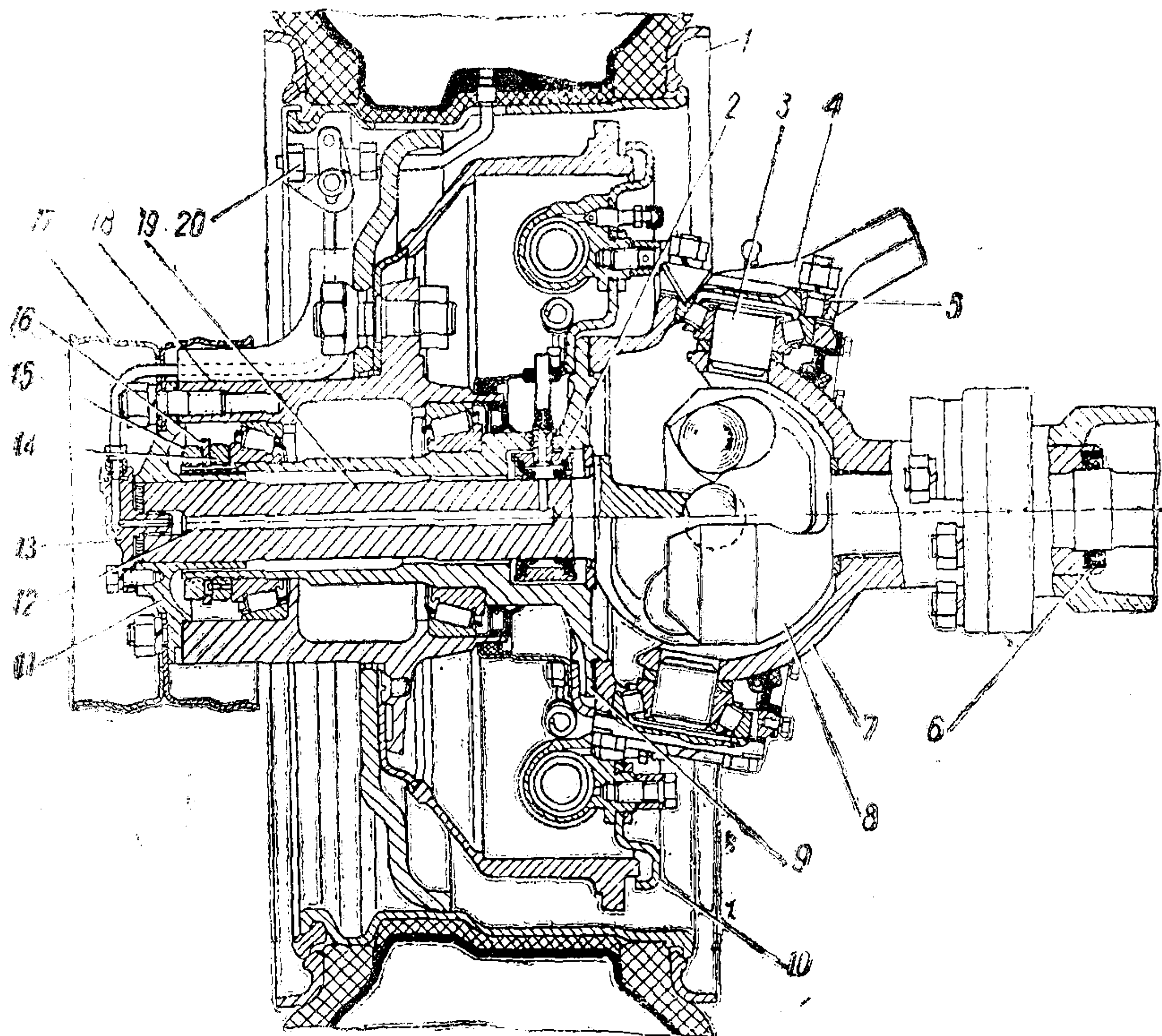
Рис. 29. Привод к передним колесам автомобиля:
