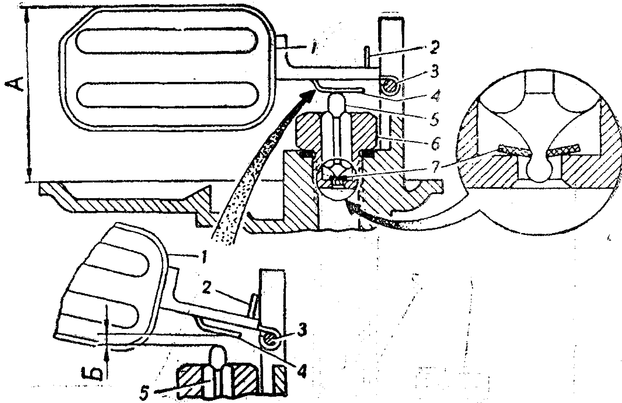
Рис. 85. Поплавковый механизм карбюратора:
