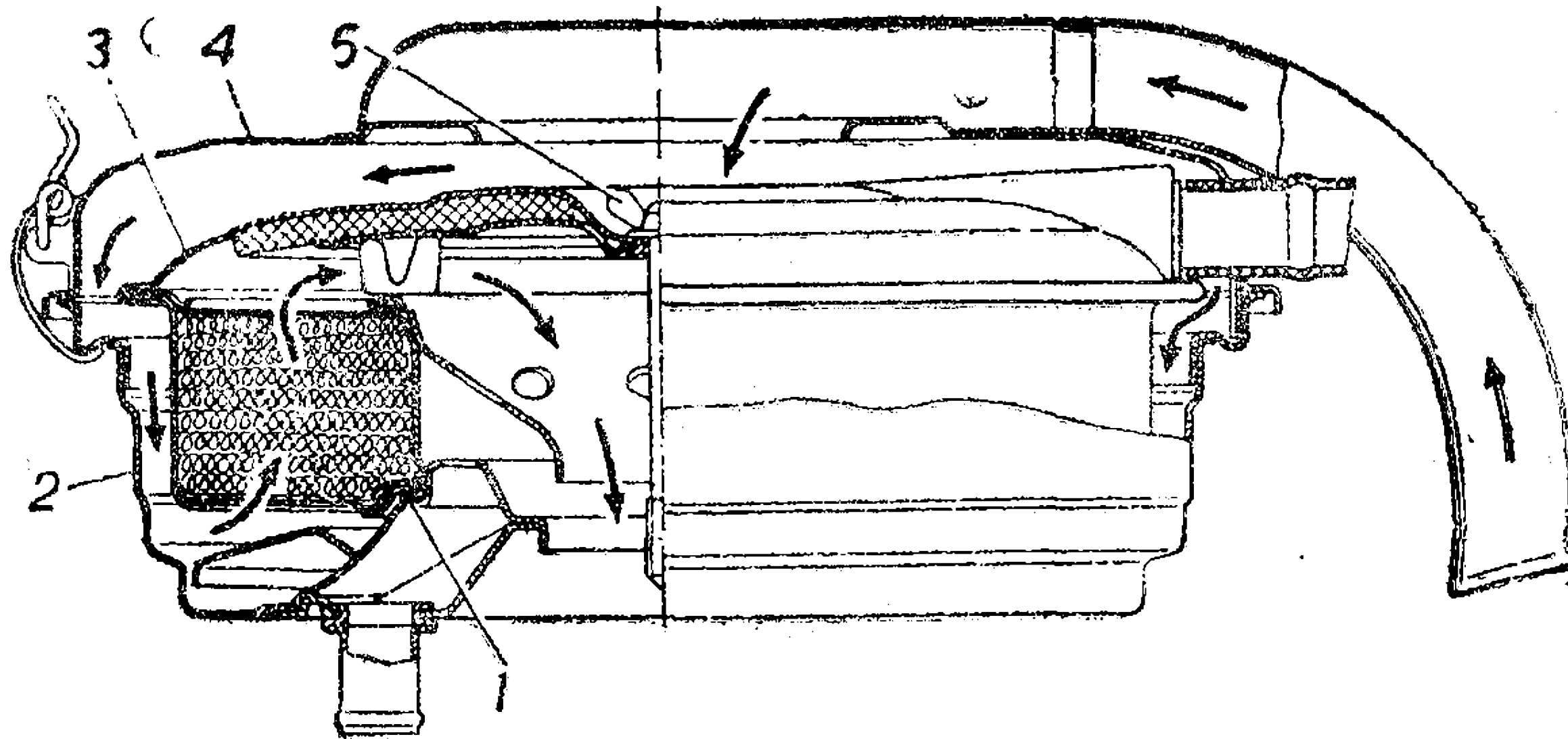
Рис. 19. Воздушный фильтр:
