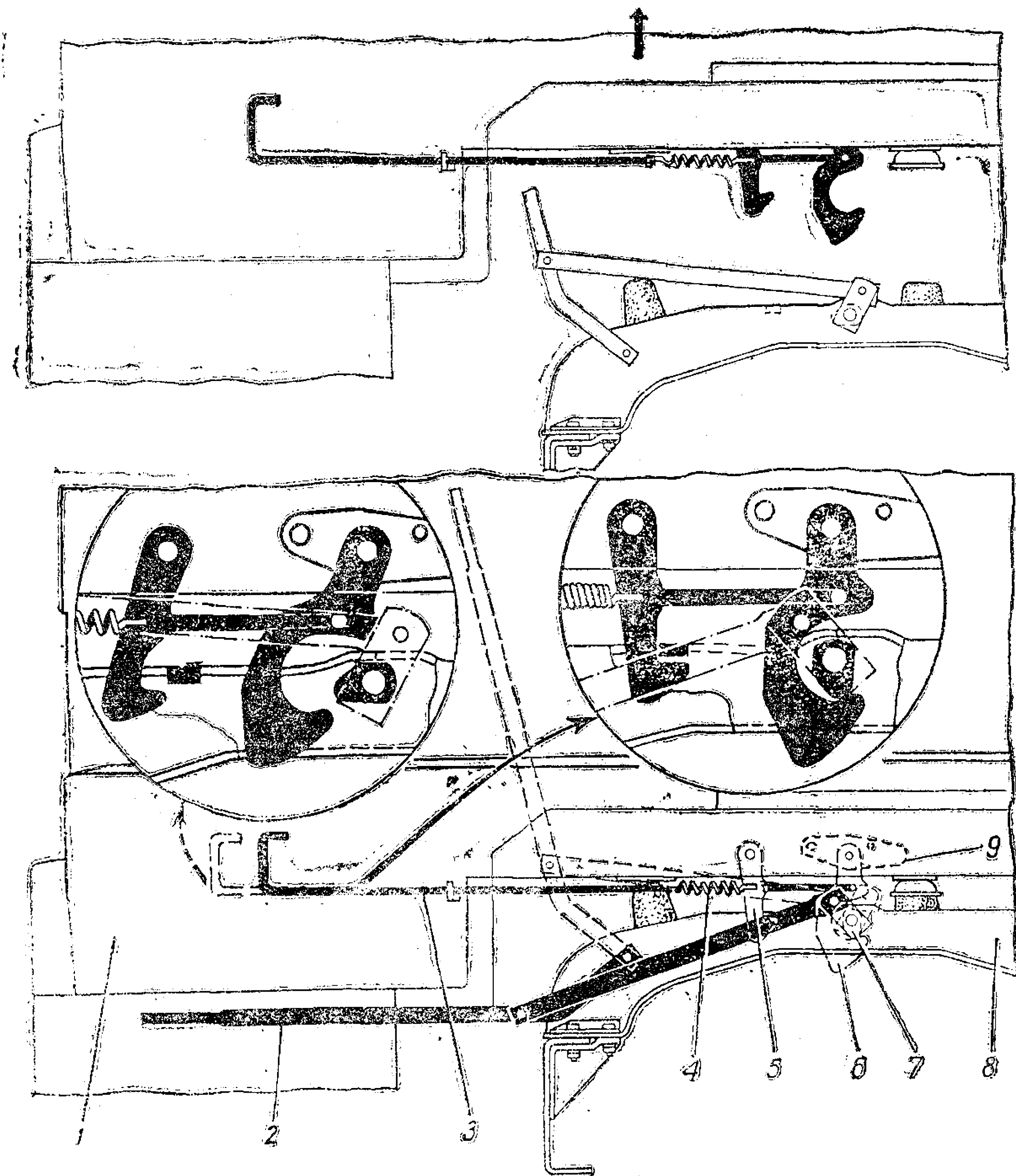
Рис. 70. Запорный механизм кабины:
