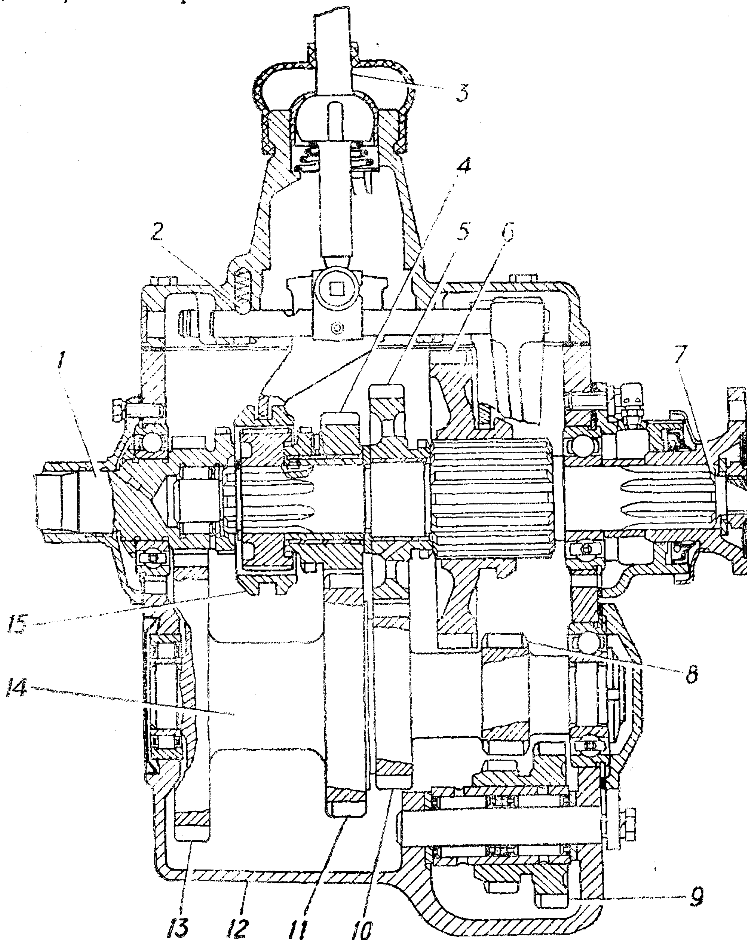
Рис. 26. Коробка передач:
