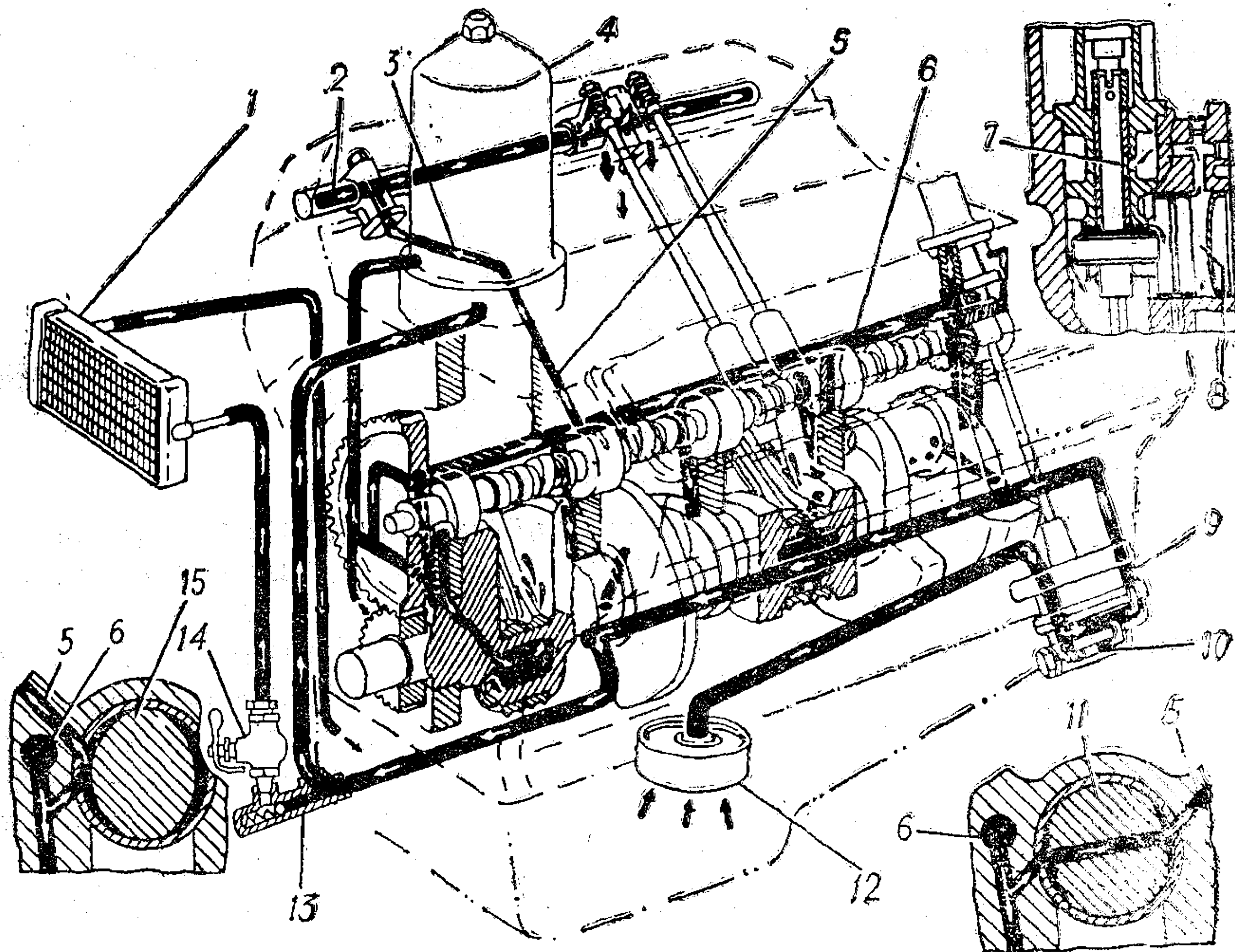
Рис. 11. Схема смазки двигателя:
