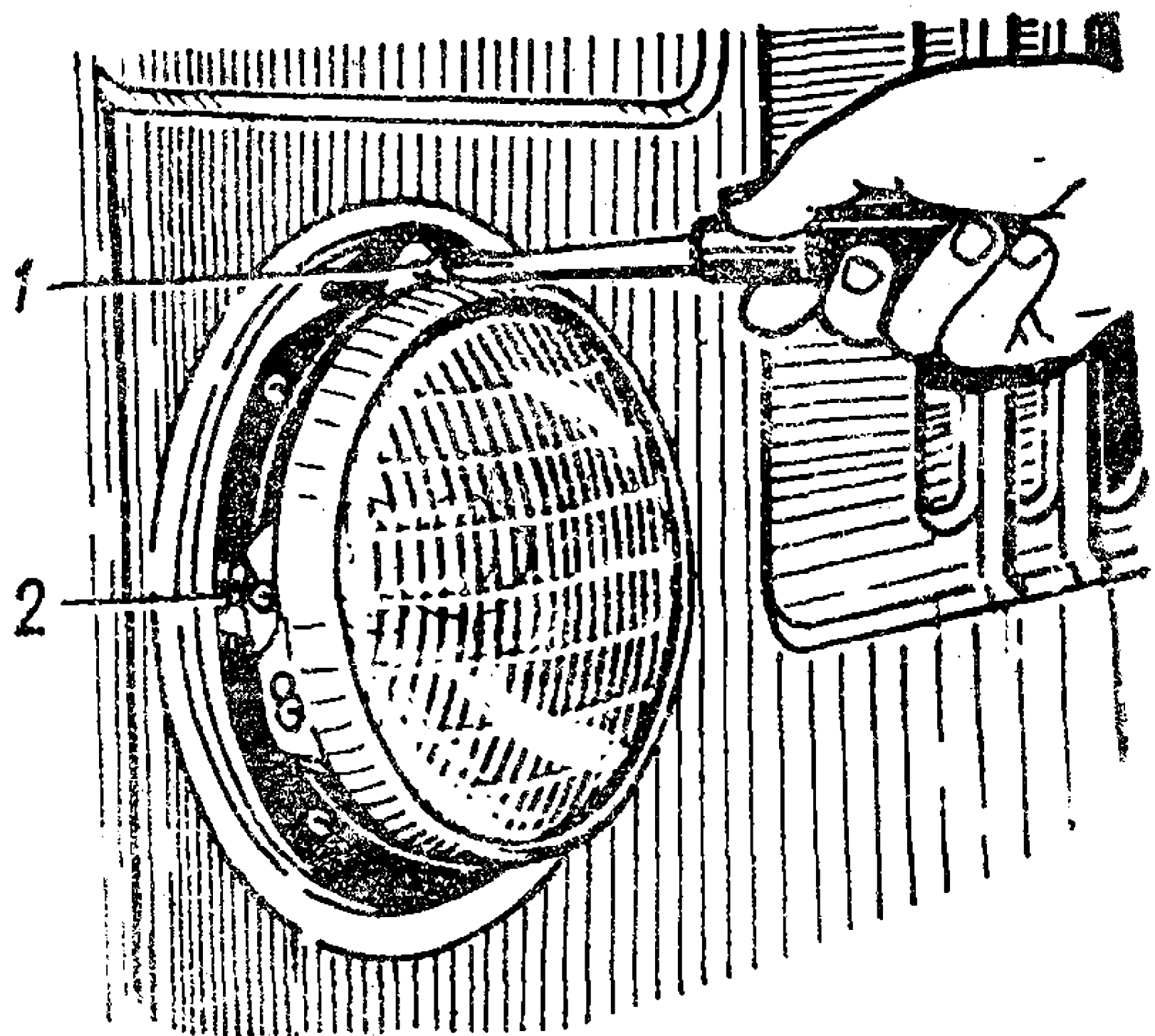
Рис. 100. Регулировка установки фар:
