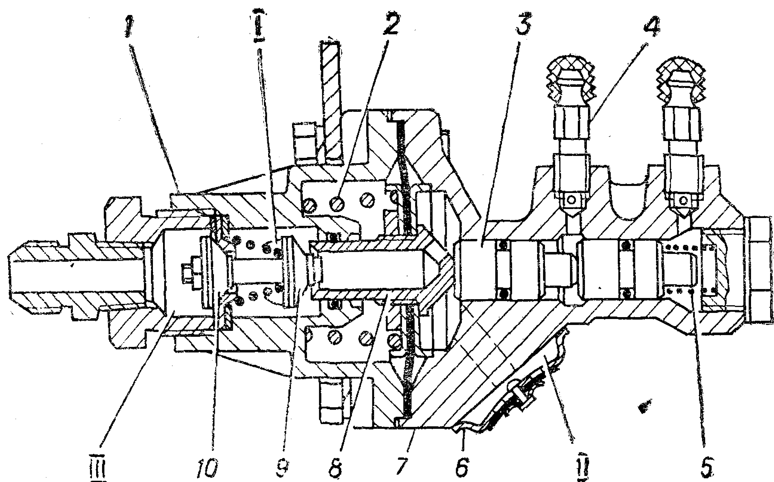
Рис. 54. Клапан управления тормозами прицепа:
