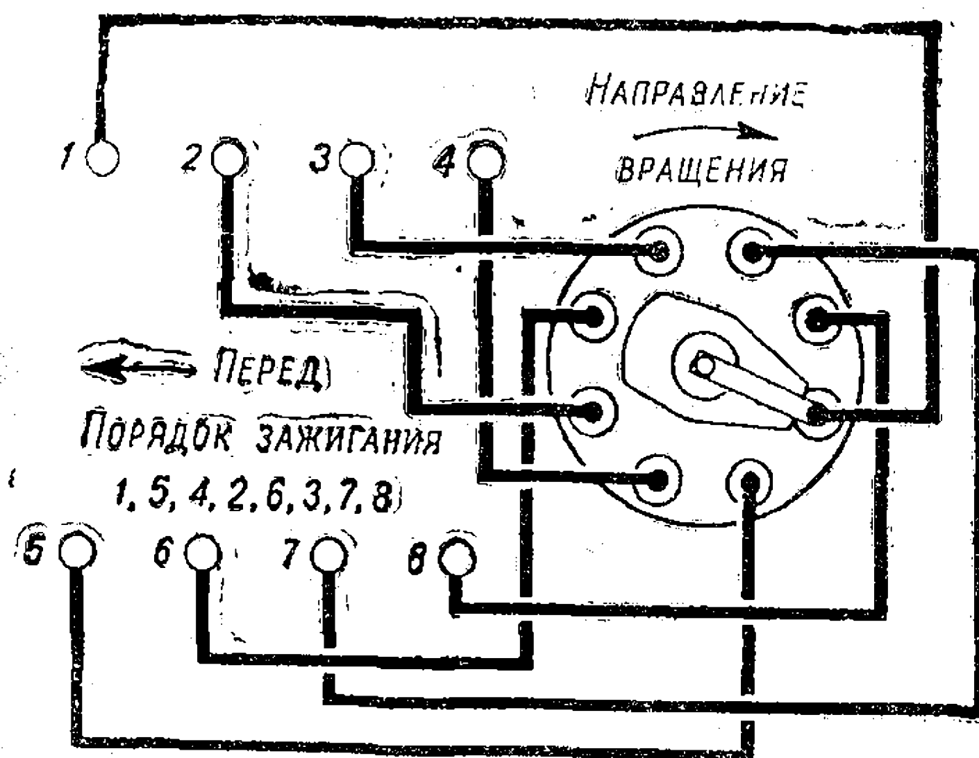
Рис. 61. Соединение проводов от датчика-распределителя к свечам
