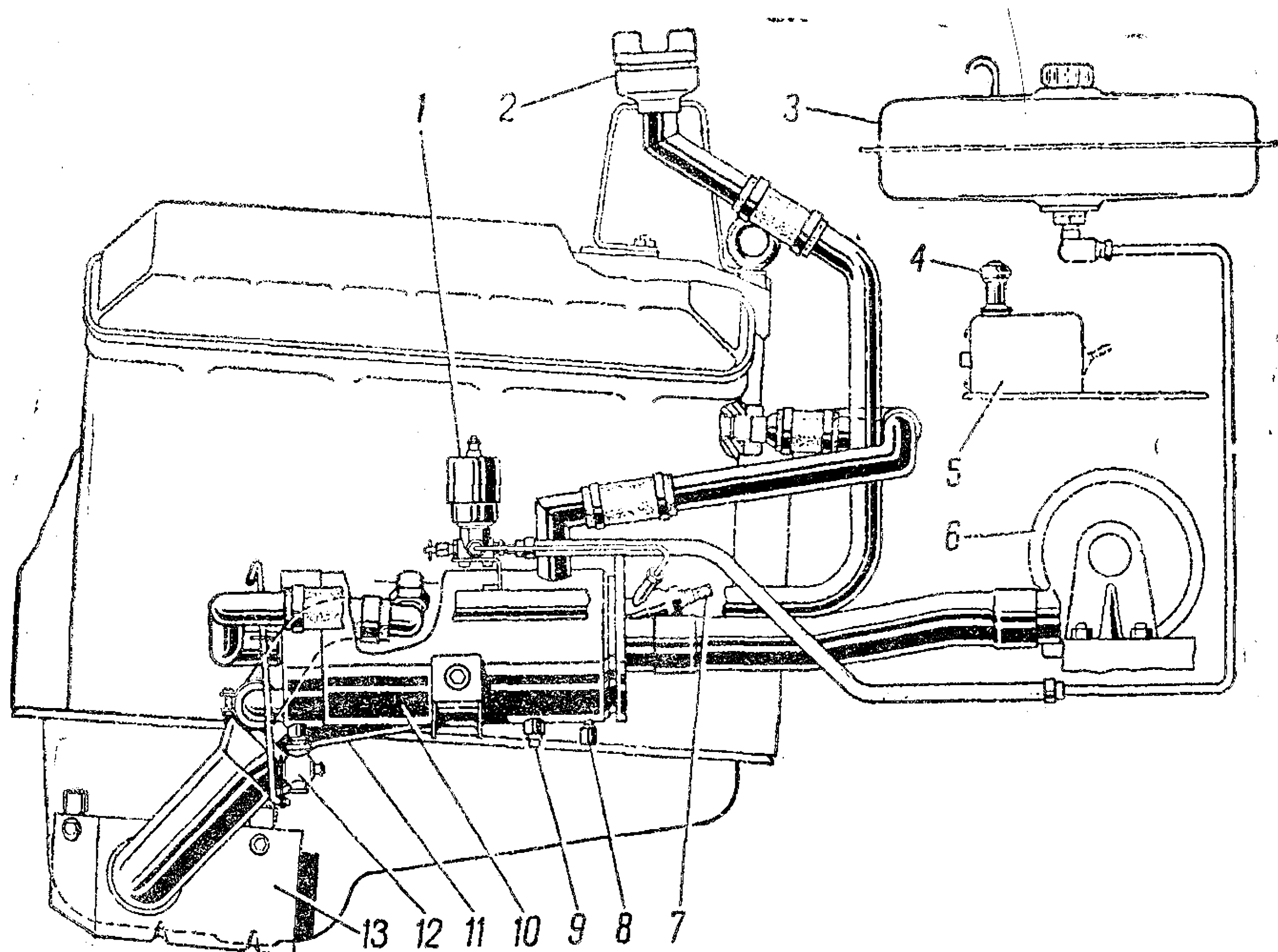
Рис. 21. Установка пускового оборудования:
