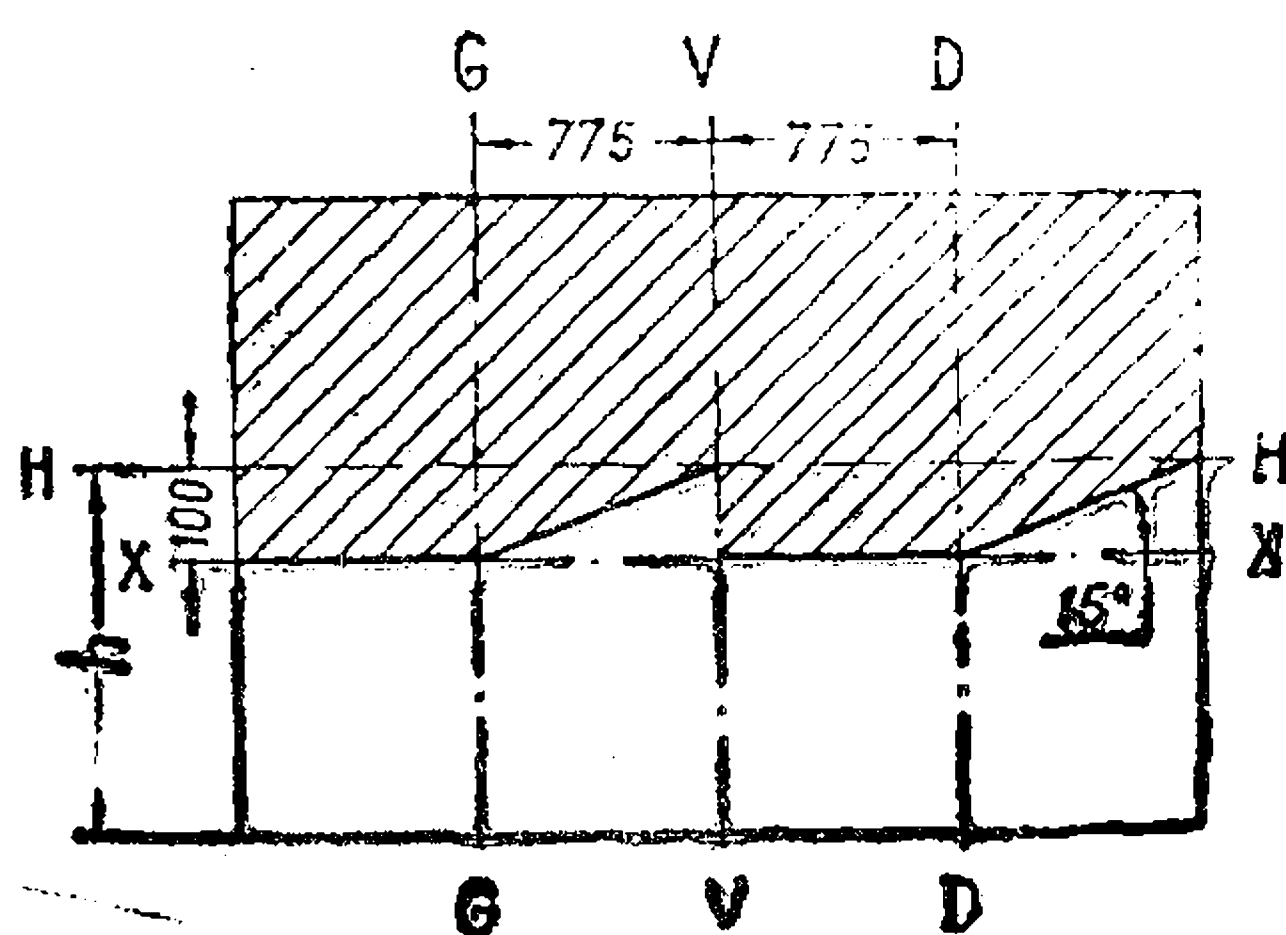
Рис. 99. Разметка экрана для регулировки фар: h—высота от земли (пола) до центра фар
