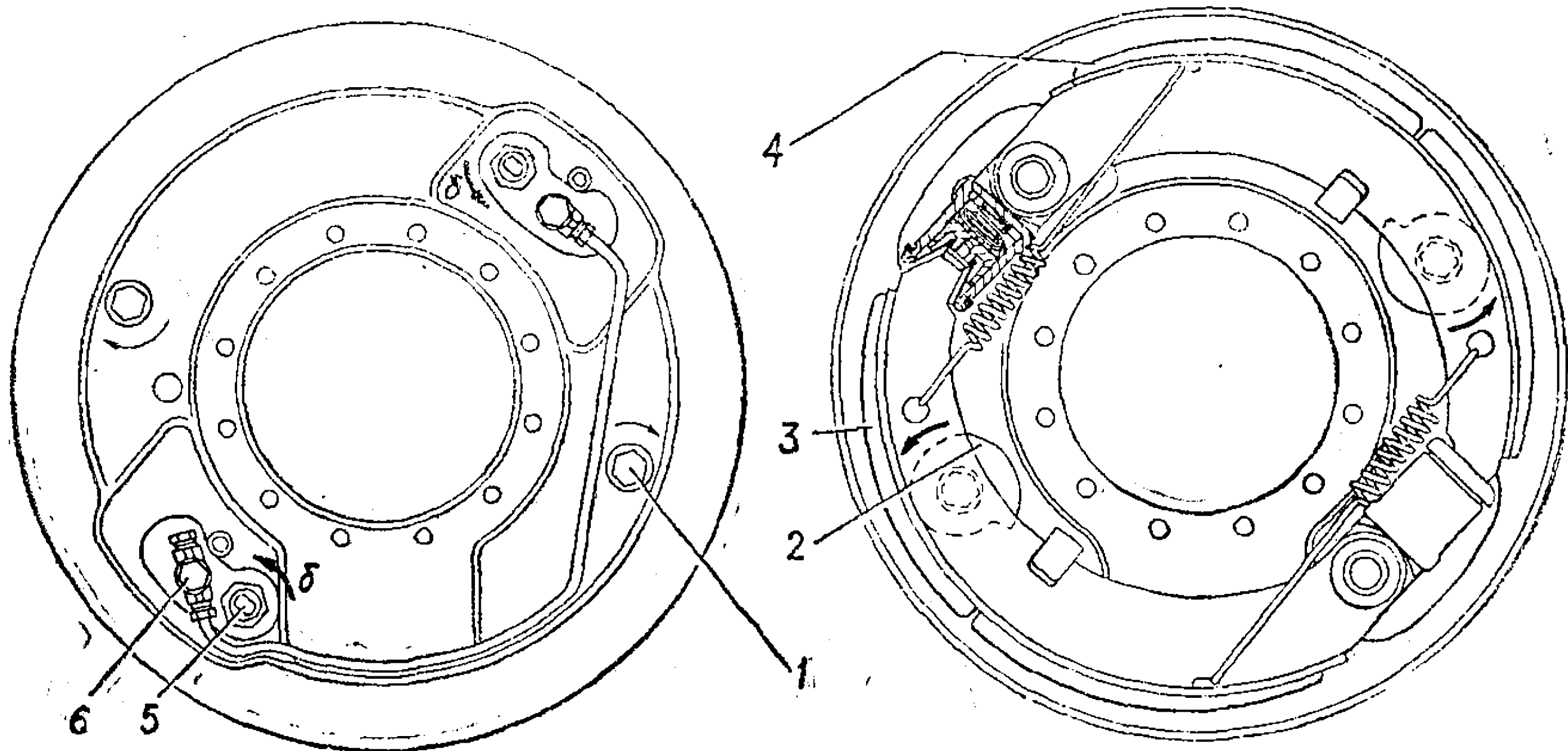
Рис. 95. Рабочий тормоз передних колес:
