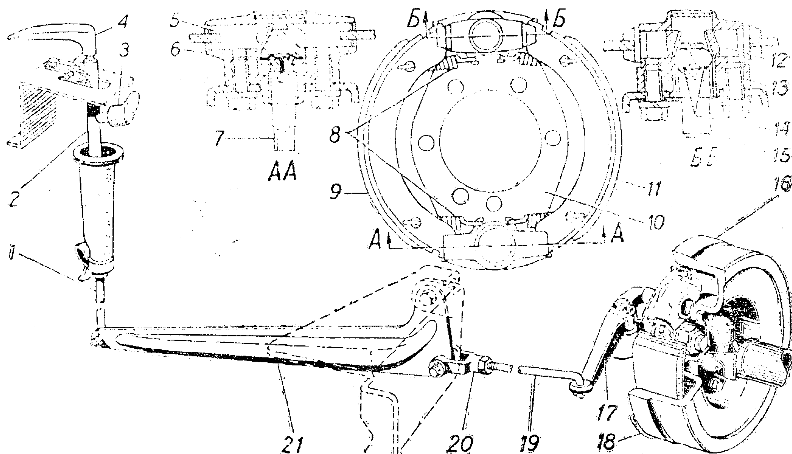
Рис. 98. Стояночная тормозная система:
