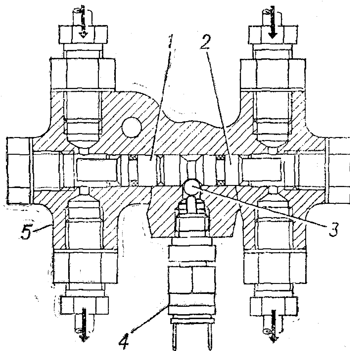
Рис. 53. Сигнальное устройство:
