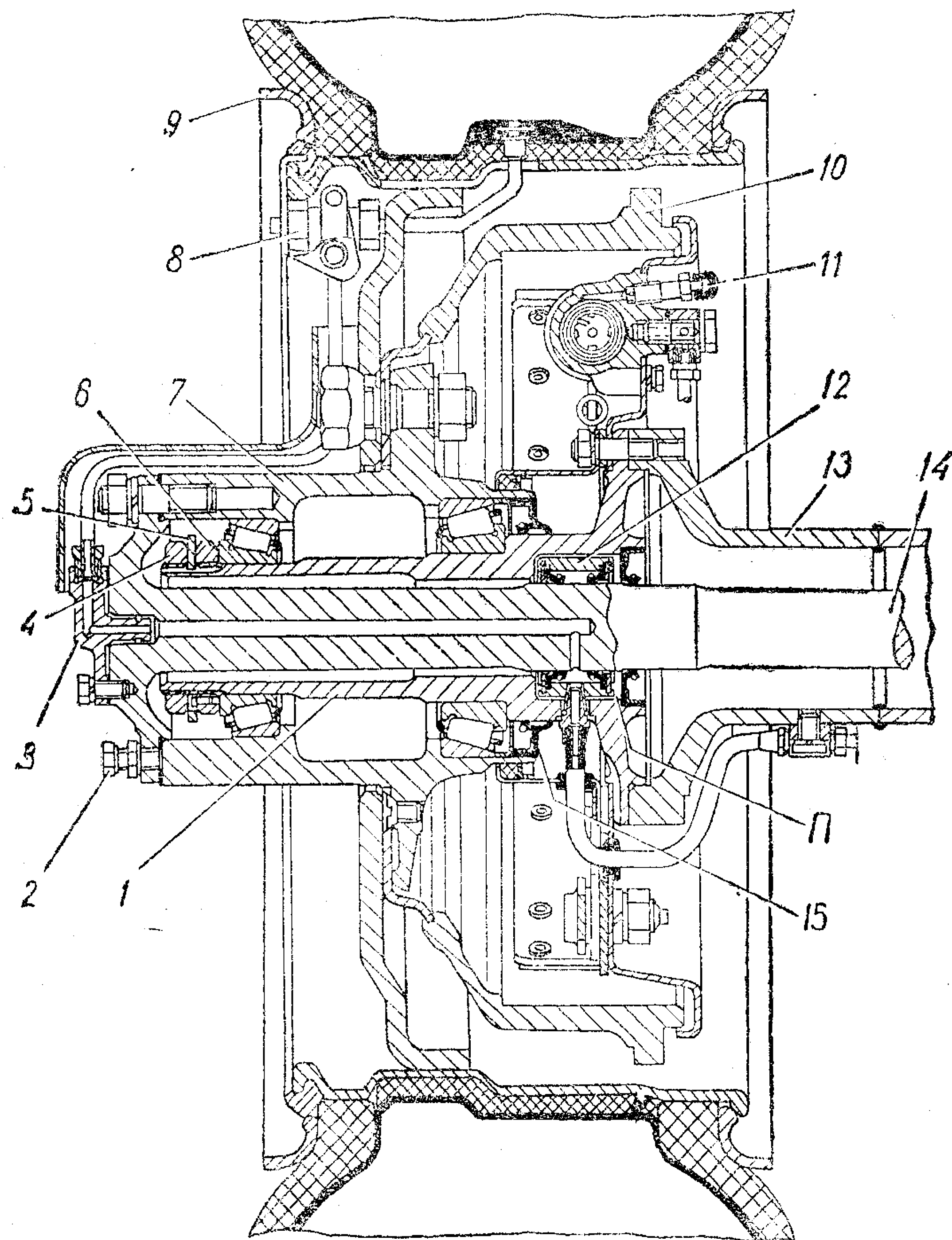
Рис. 90. Задняя ступица и колесо:
