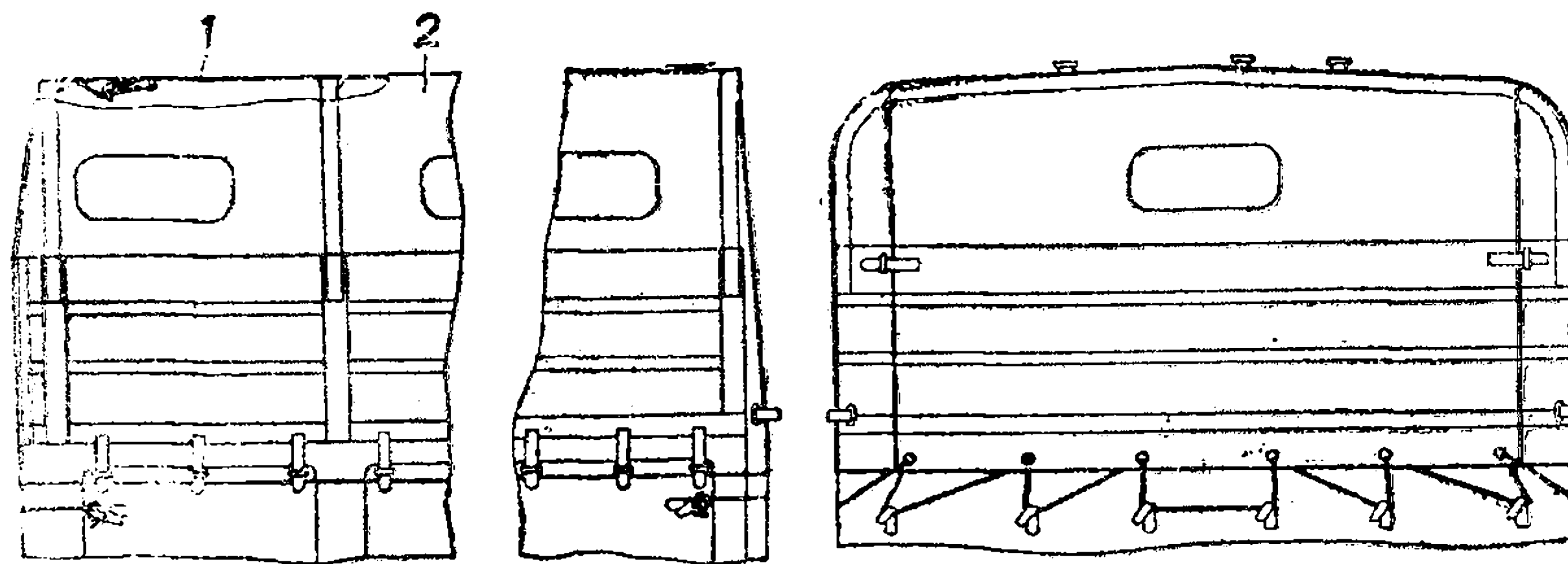
Рис. 77. Установка тента на платформу:
