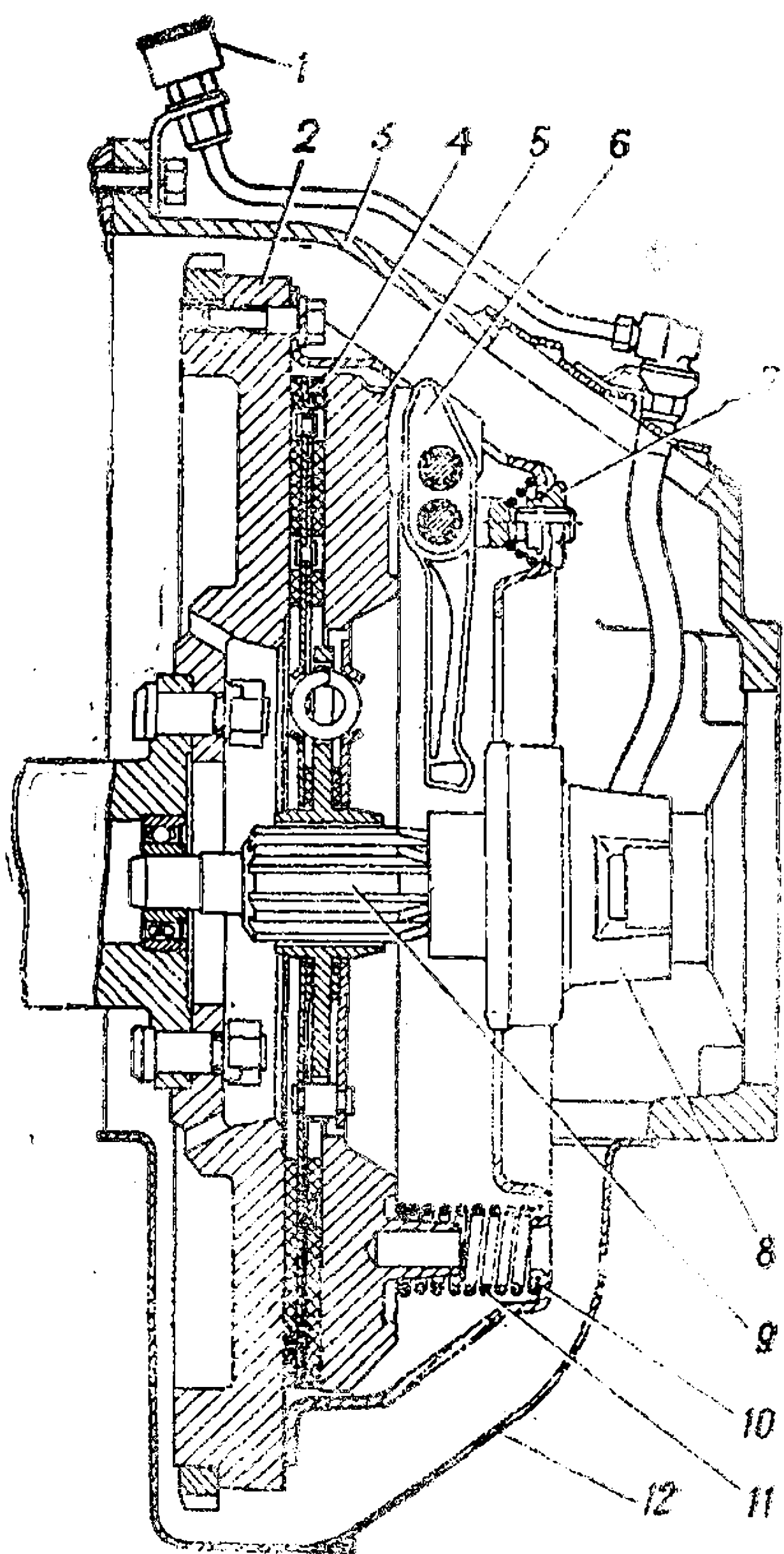
Рис. 24. Сцепление:
