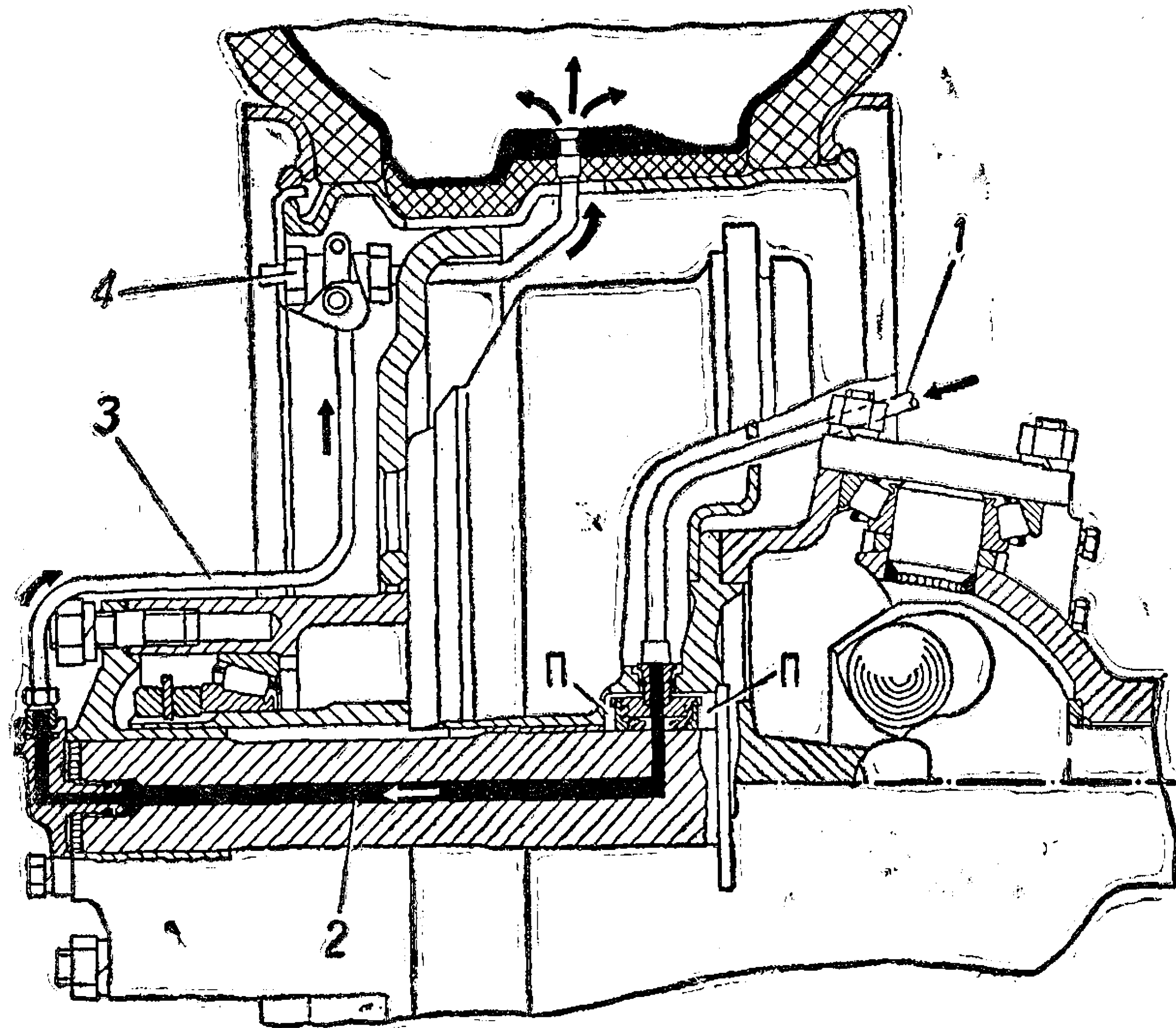
Рис. 44. Подвод воздуха к переднему колесу:
