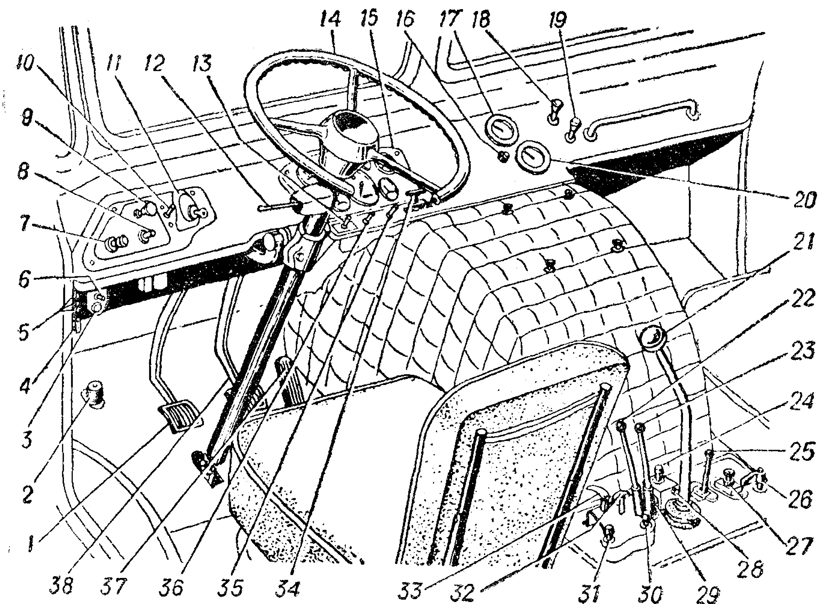
Рис. 1. Расположение органов управления автомобилем:
