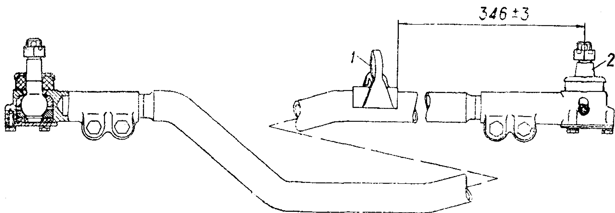
Рис. 93. Поперечная рулевая тяга автомобиля:
