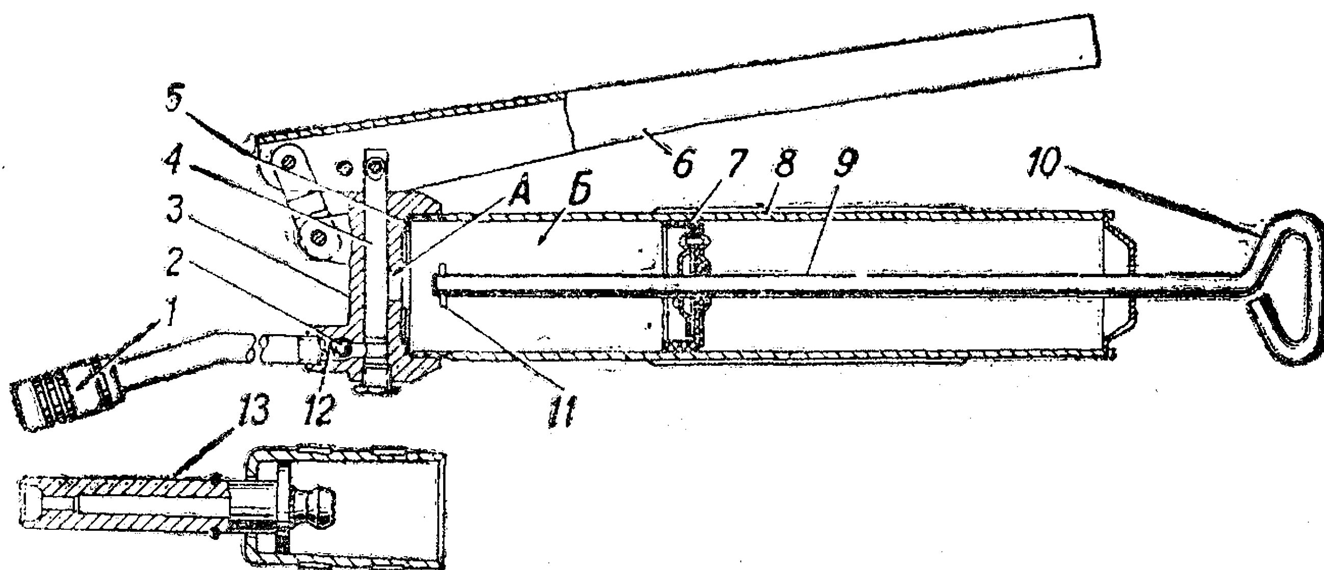
Рис. 81. Рычажно-плунжерный шприц:
