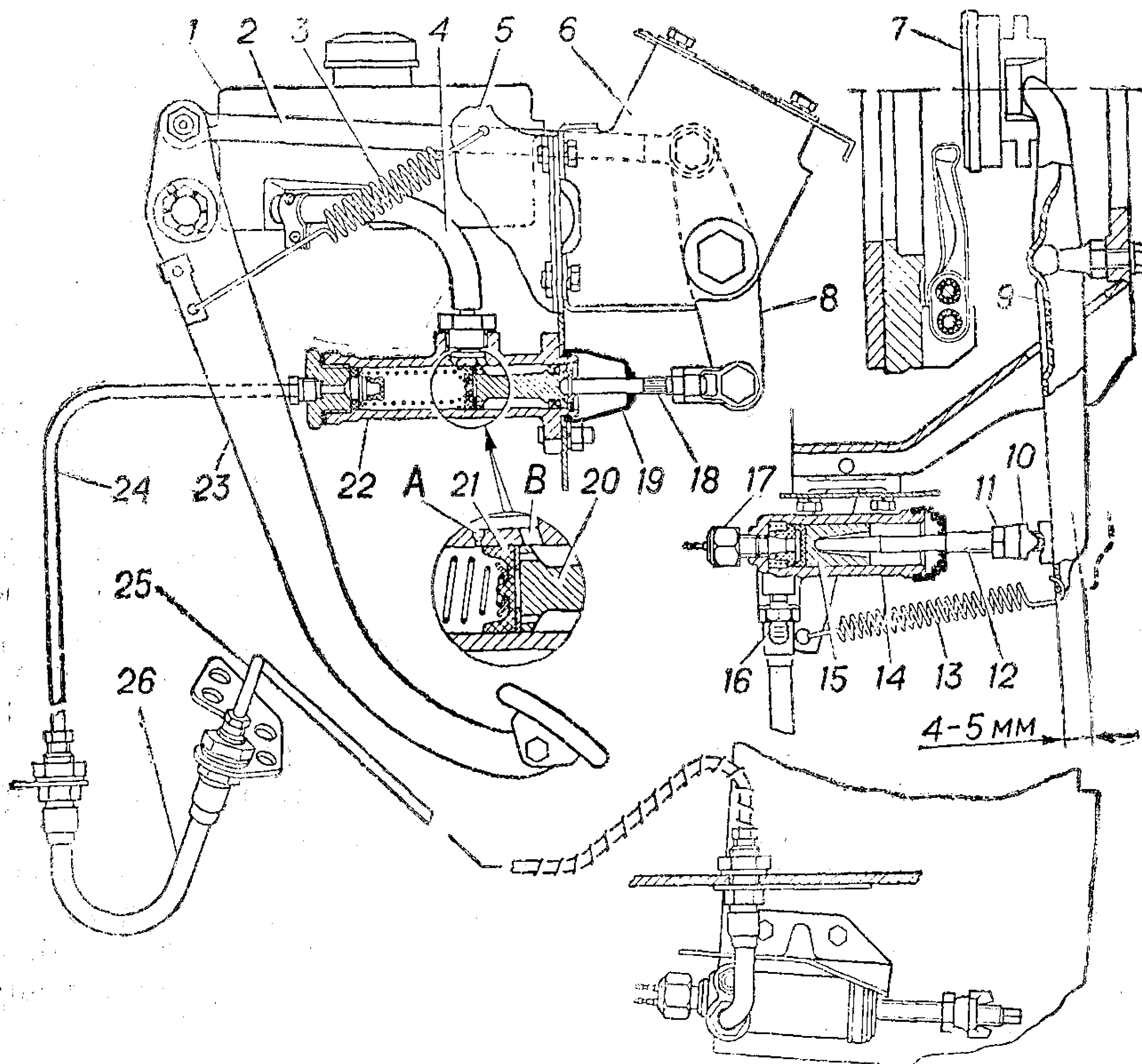
Рис. 25. Привод сцепления:
