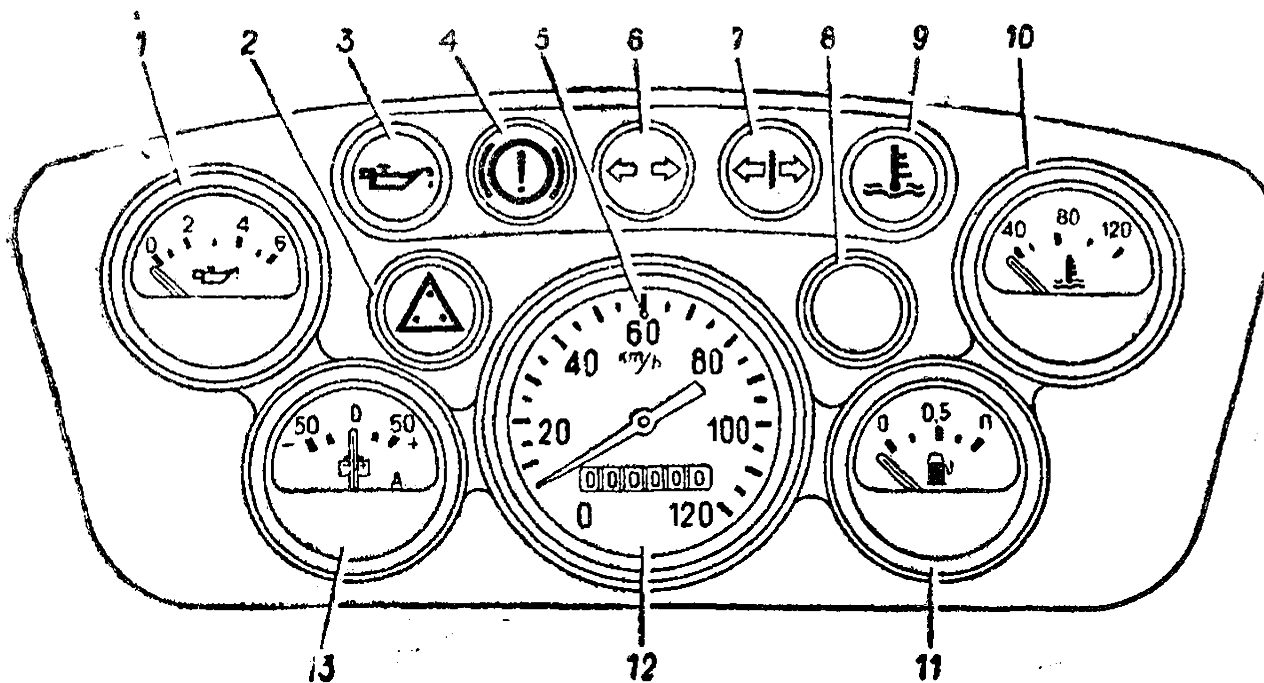
Рис. 3. Щиток приборов:
