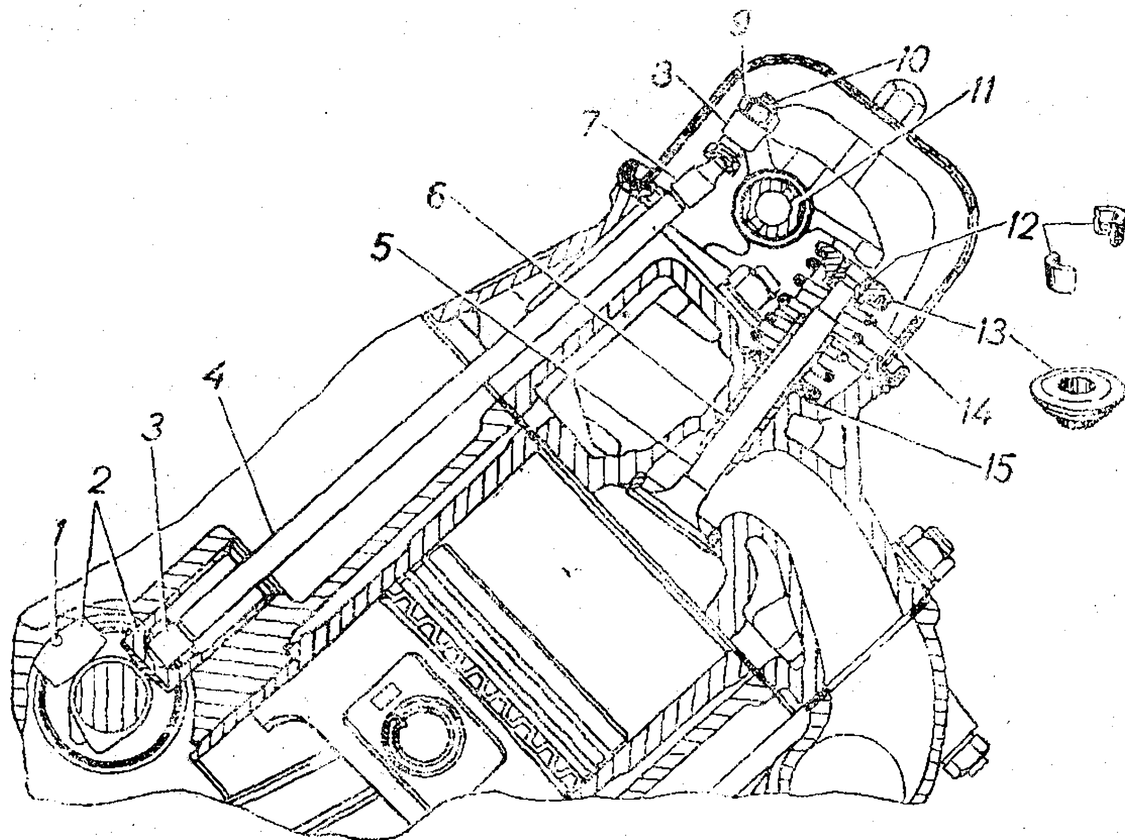
Рис. 10. Механизм привода клапанов:
