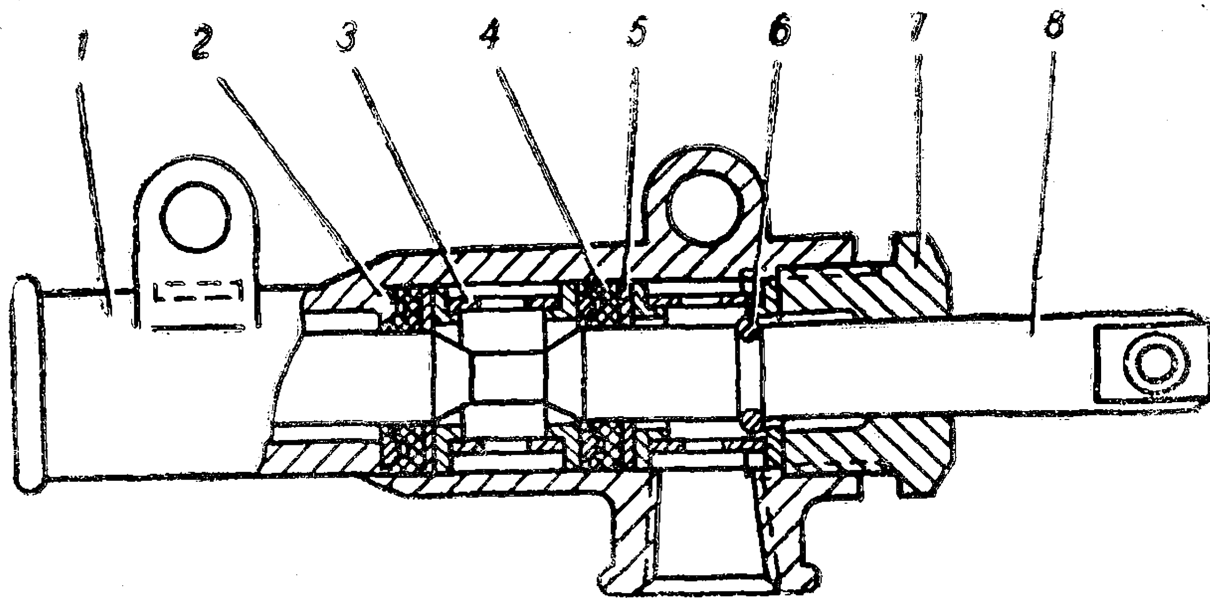
Рис. 42. Кран управления:
