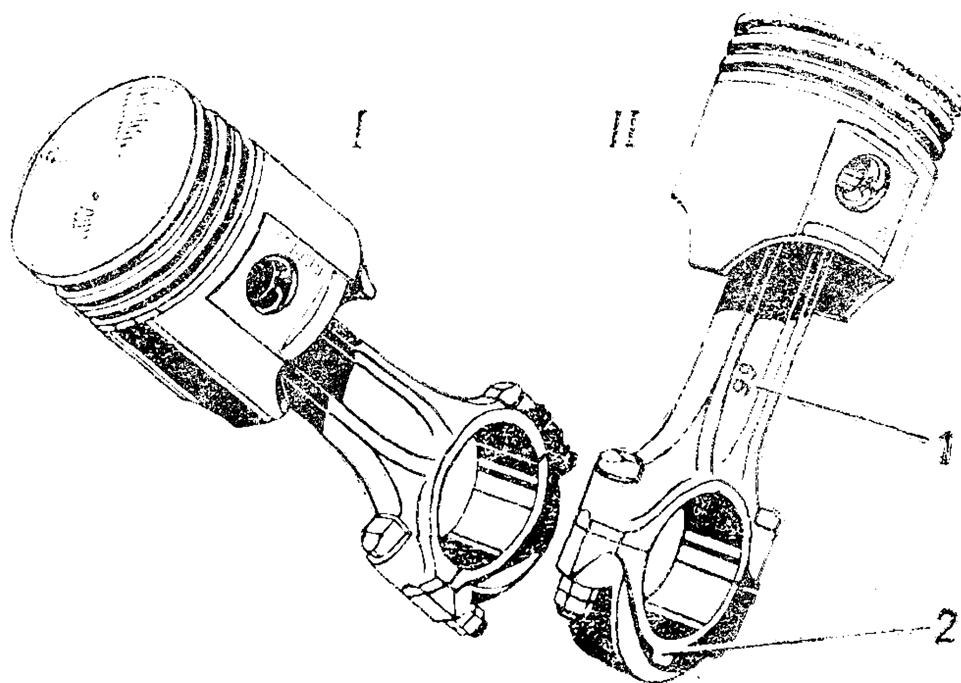
Рис. 9. Соединение шатуна с поршнем:
