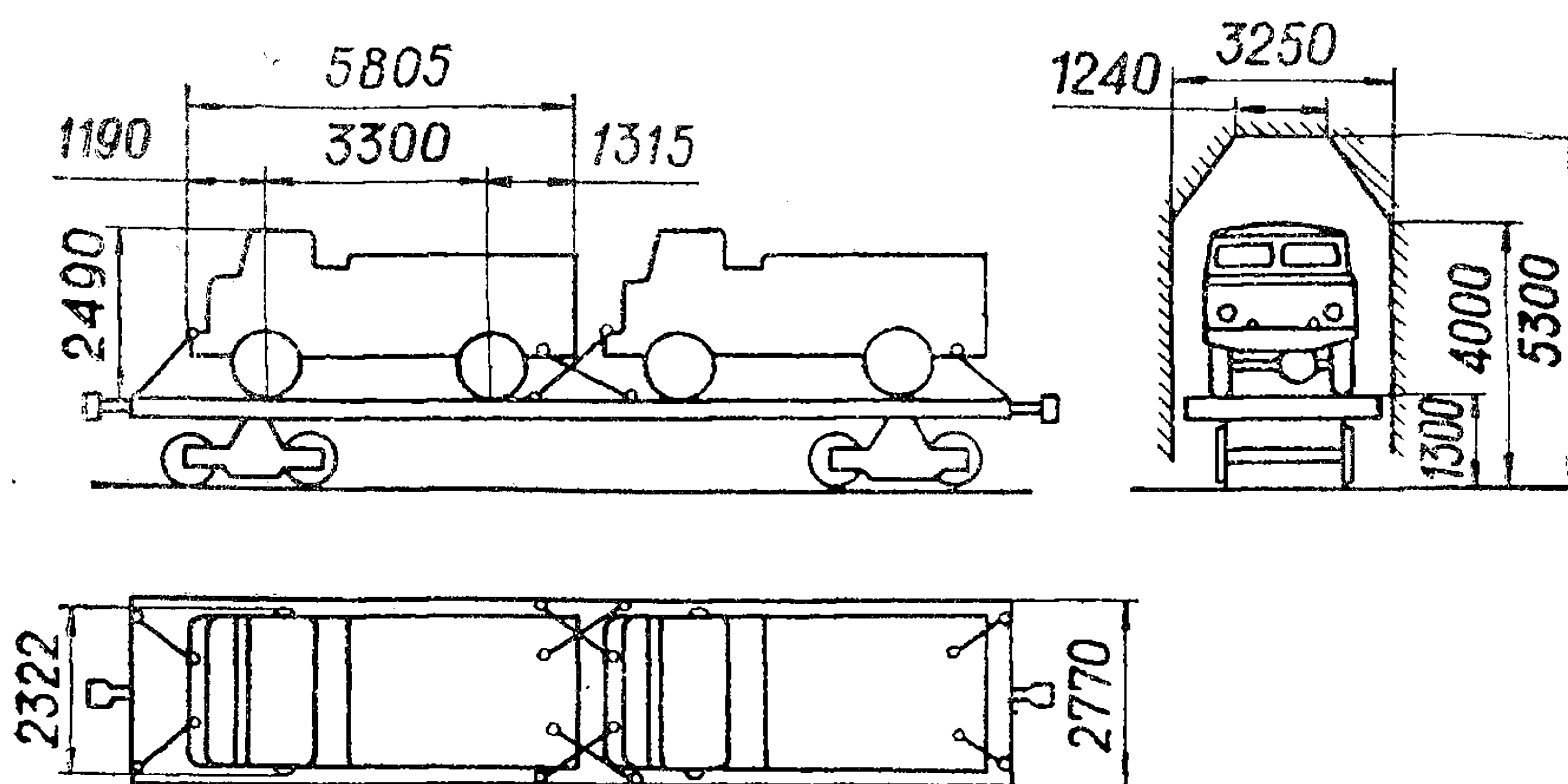
Рис. 102. Схема погрузки автомобилей на железнодорожную платформу
