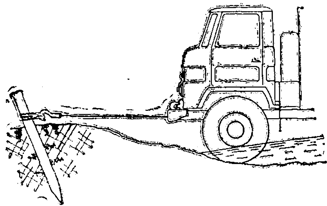
Рис. 69. Самовытаскивание автомобиля с помощью лебедки
