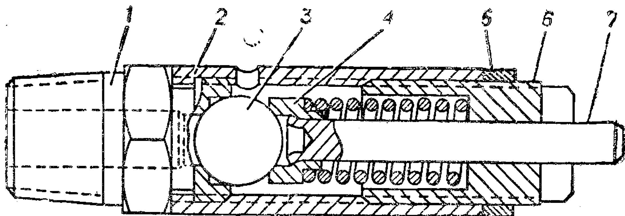
Рис. 41. Предохранительный клапан:
