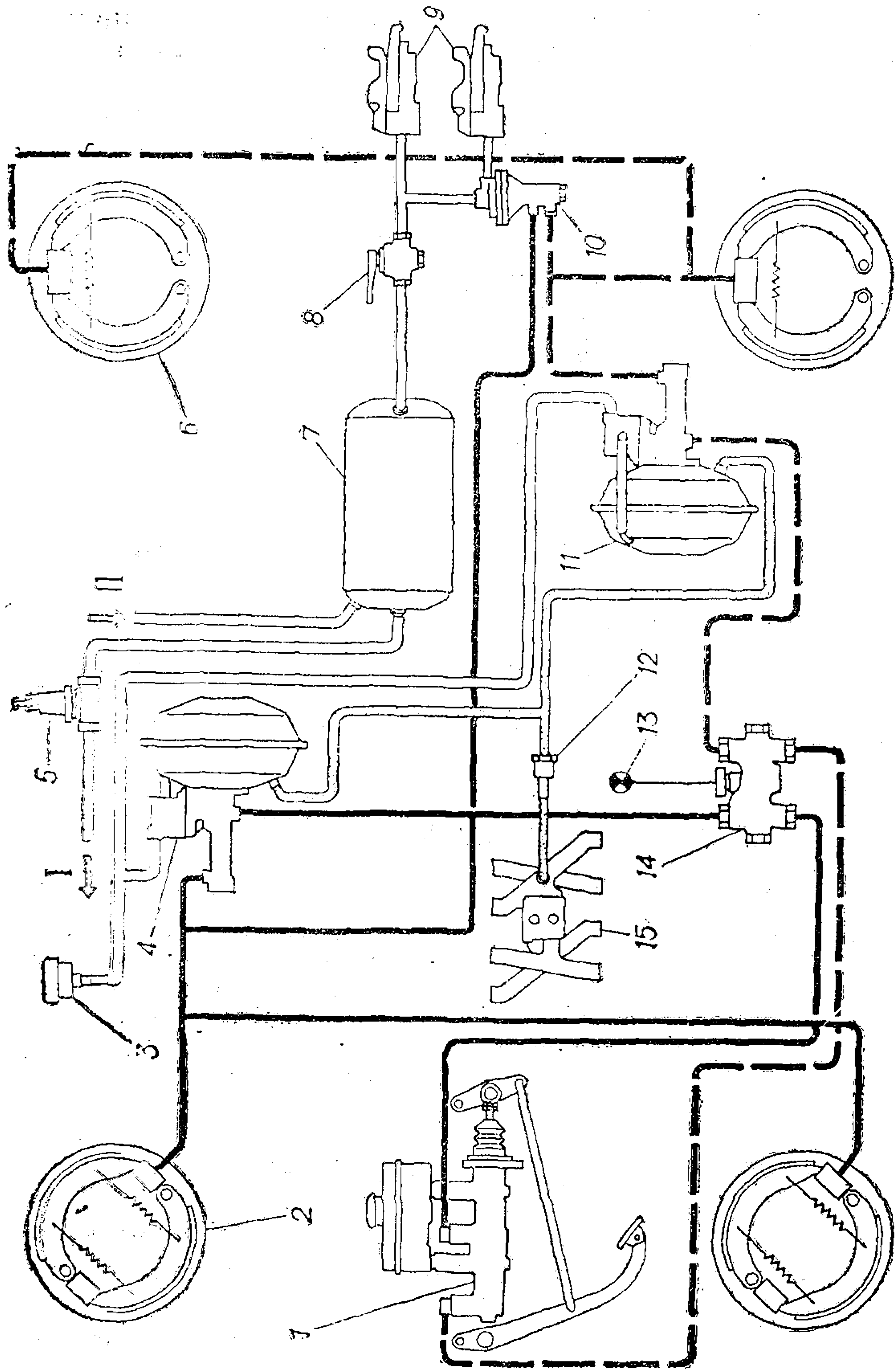
Рис. 50. Схема привода рабочей тормозной системы:
