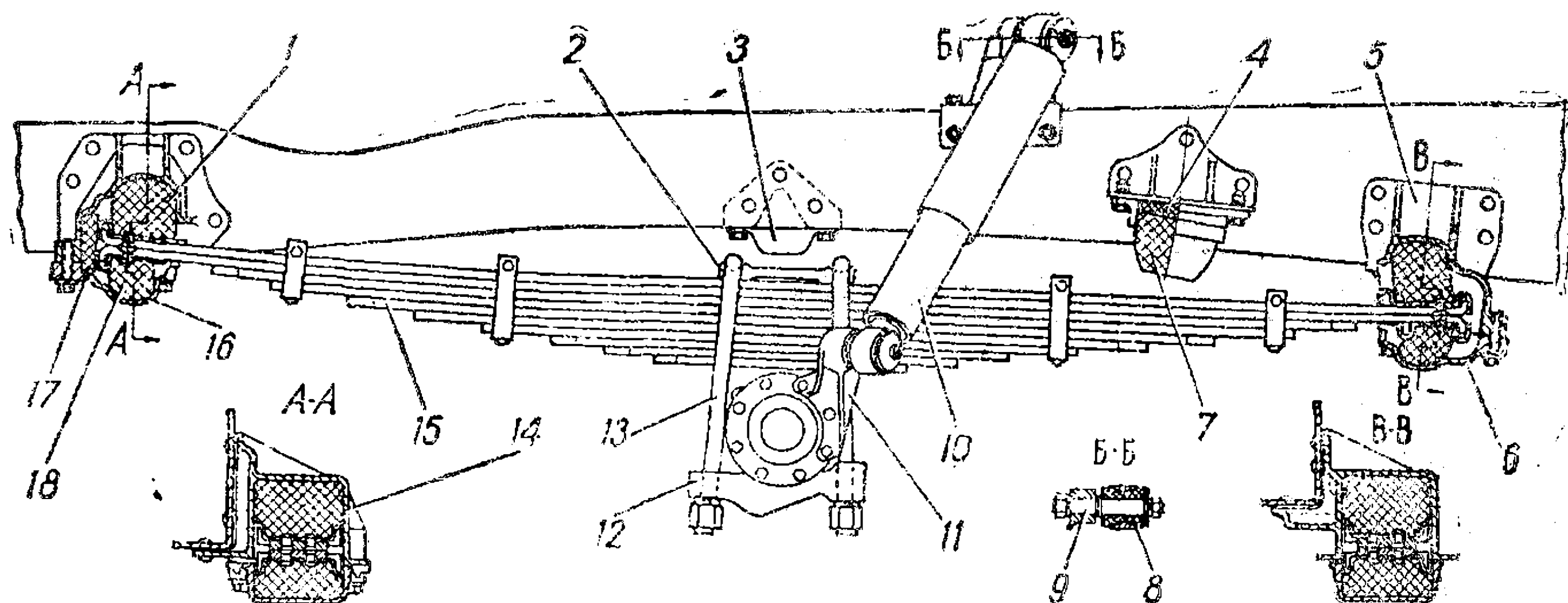
Рис. 31. Передняя подвеска
