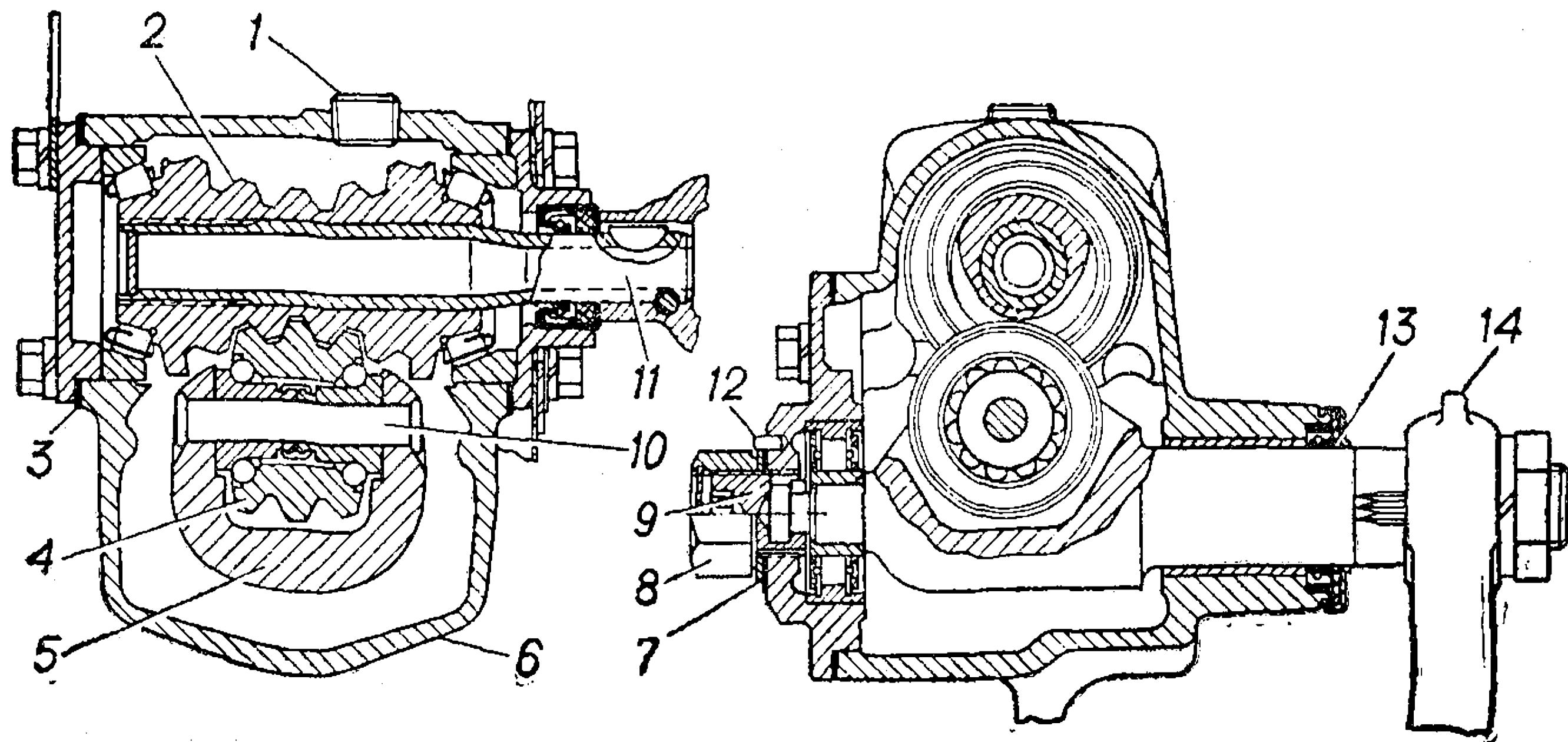
Рис. 92. Рулевой механизм:
