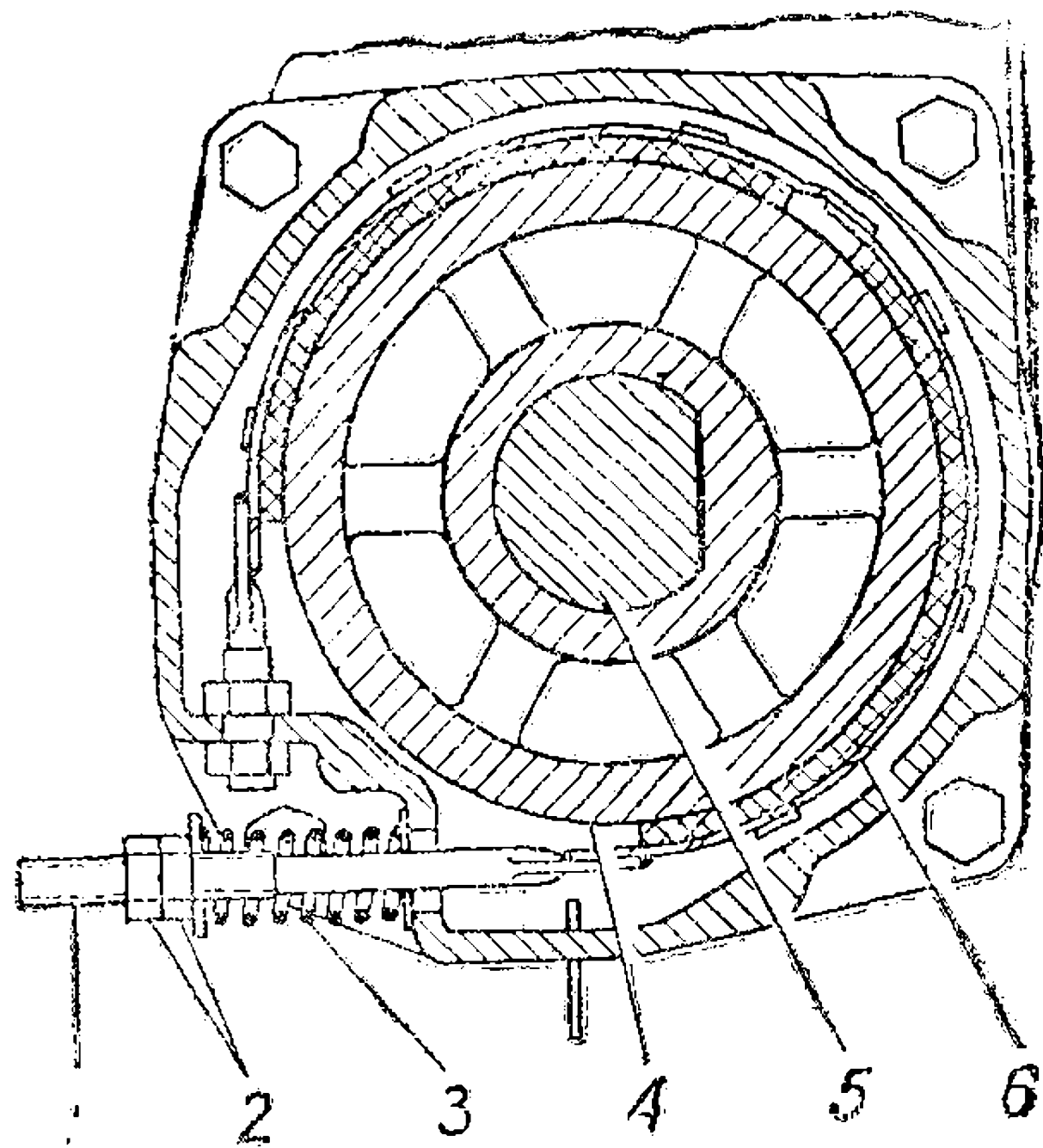
Рис. 67. Автоматический тормоз лебедки:
