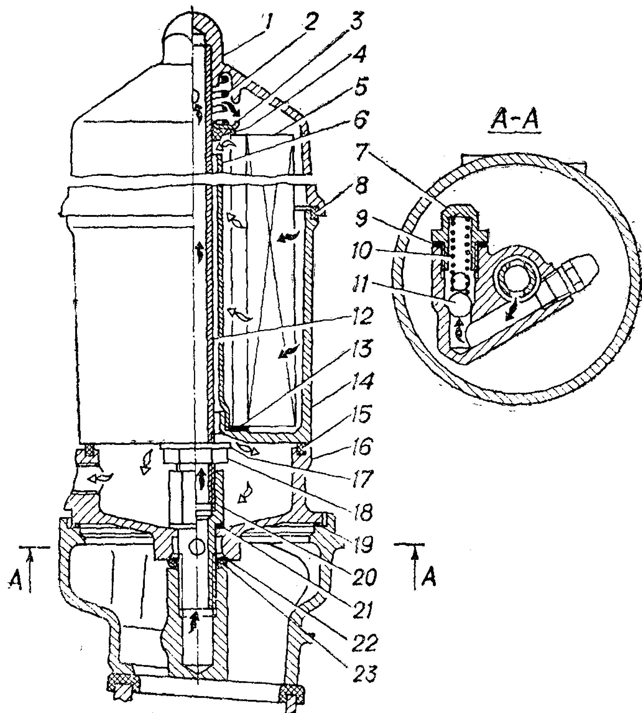
Рис. 12. Масляный фильтр:
