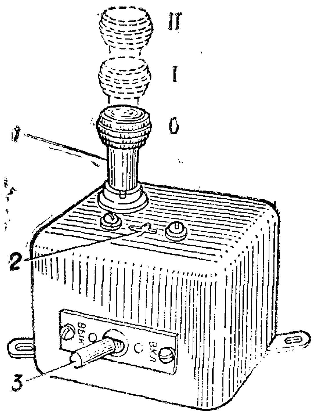
Рис. 23. Пульт управления подогревателем:
