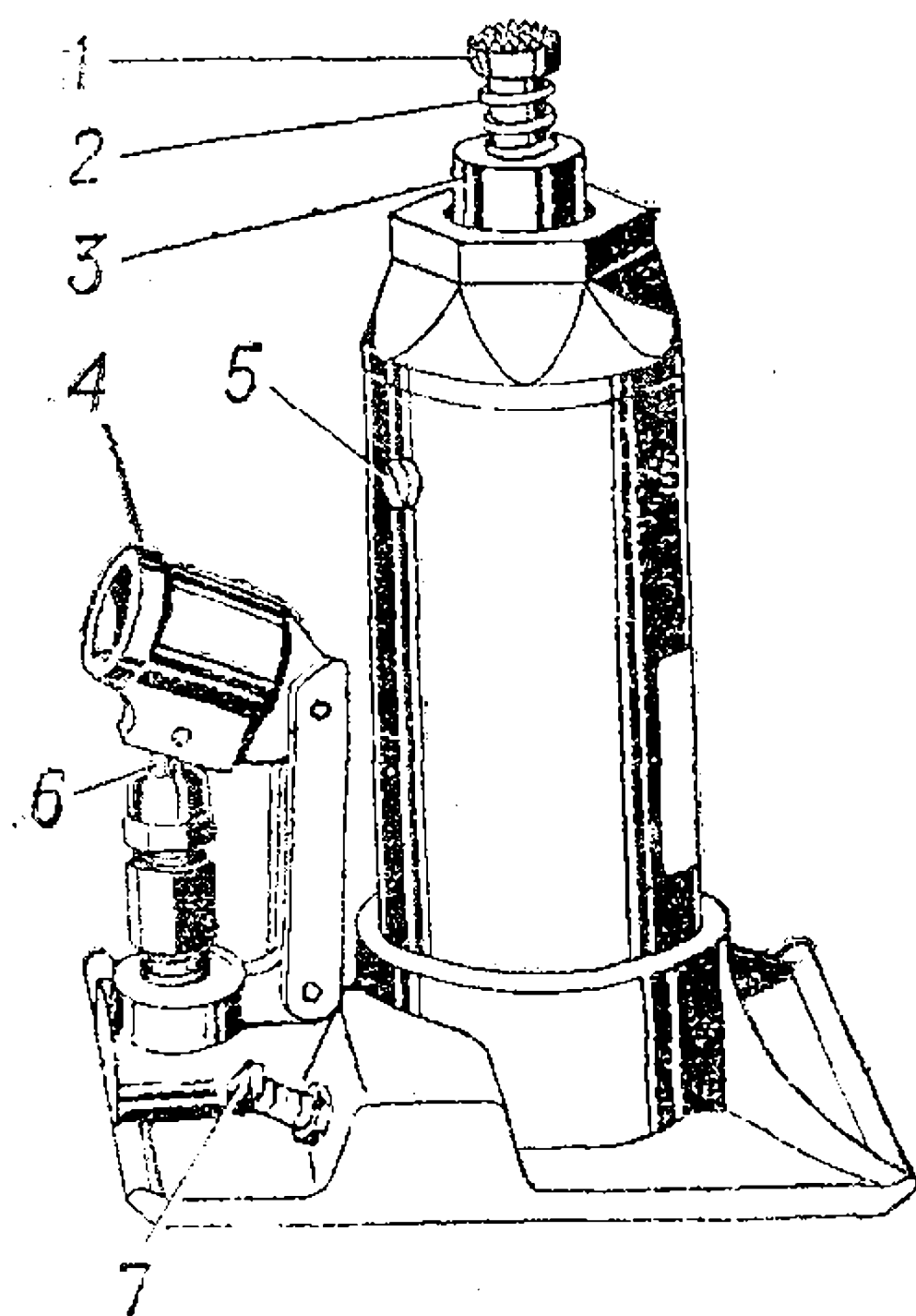
Рис. 80. Домкрат:
