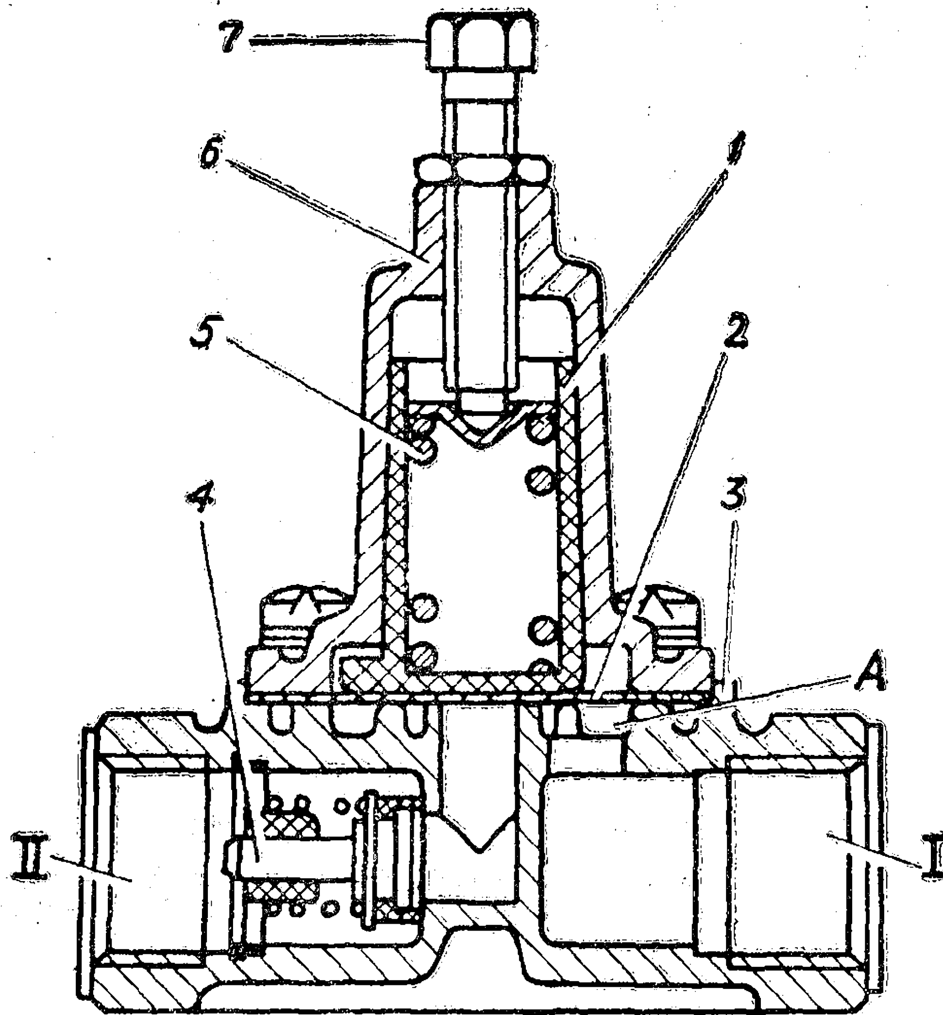
Рис. 55. Одинарный защитный клапан:
