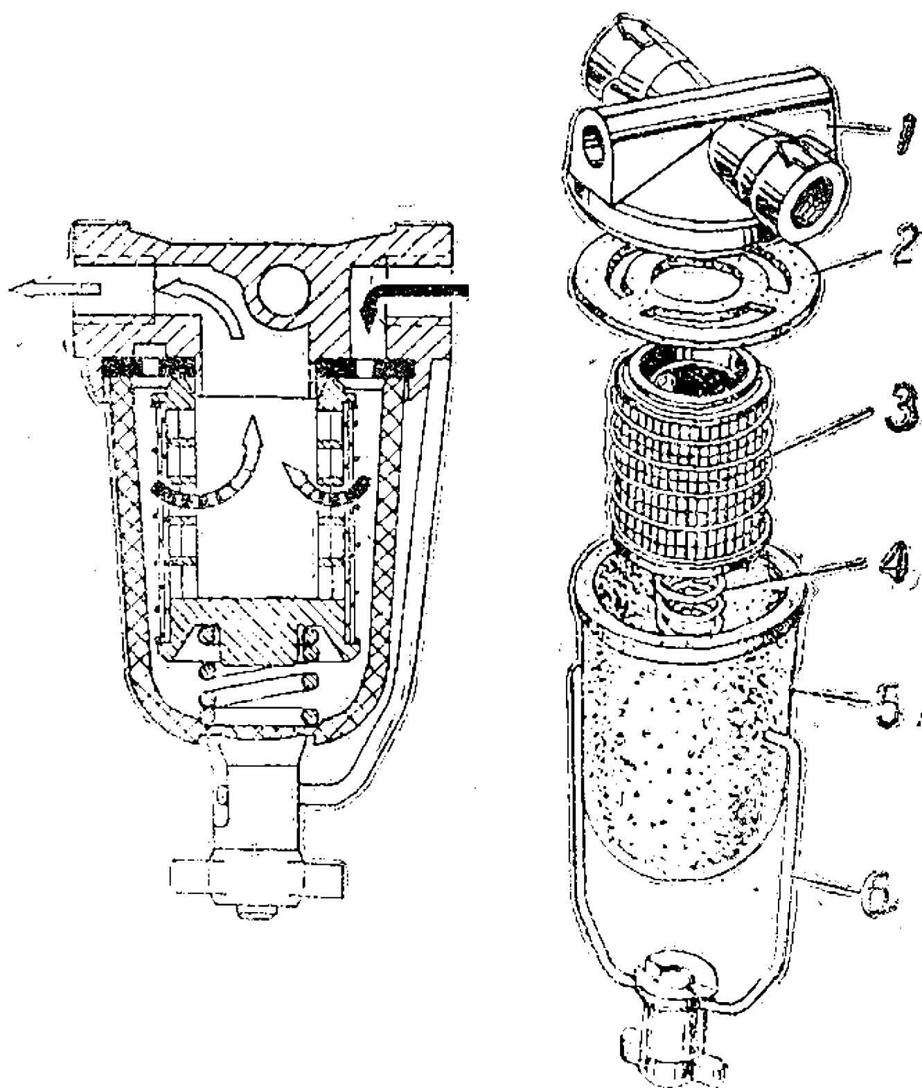
Рис. 18. Фильтр тонкой очистки бензина:
