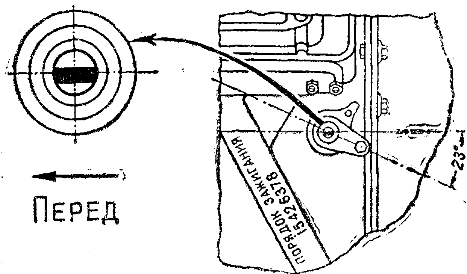
Рис. 60. Установка привода датчика-распределителя
