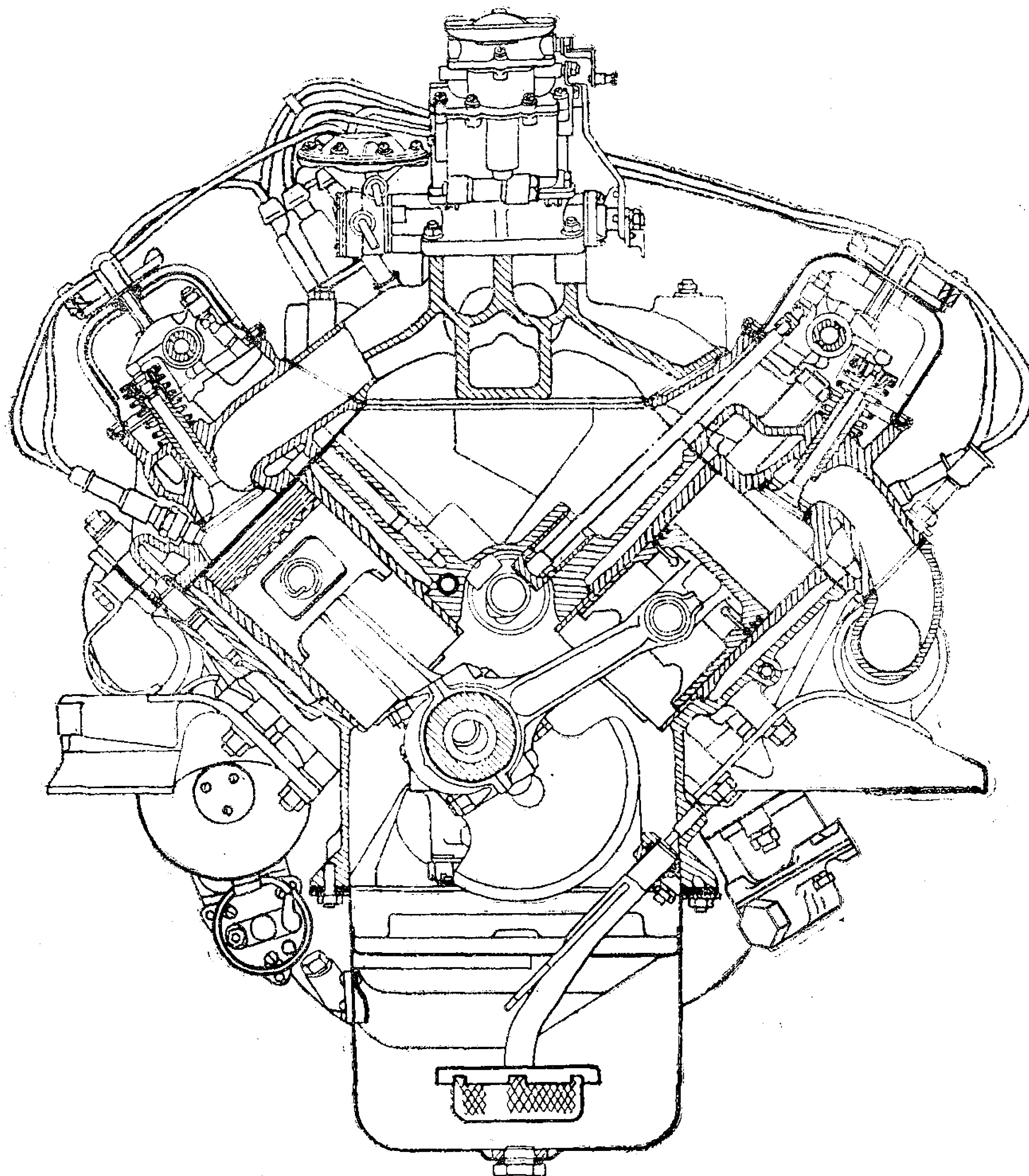
Рис. 4. Поперечный разрез двигателя
