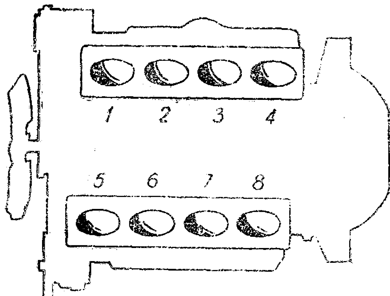
Рис. 6. Порядок нумерации цилиндров
