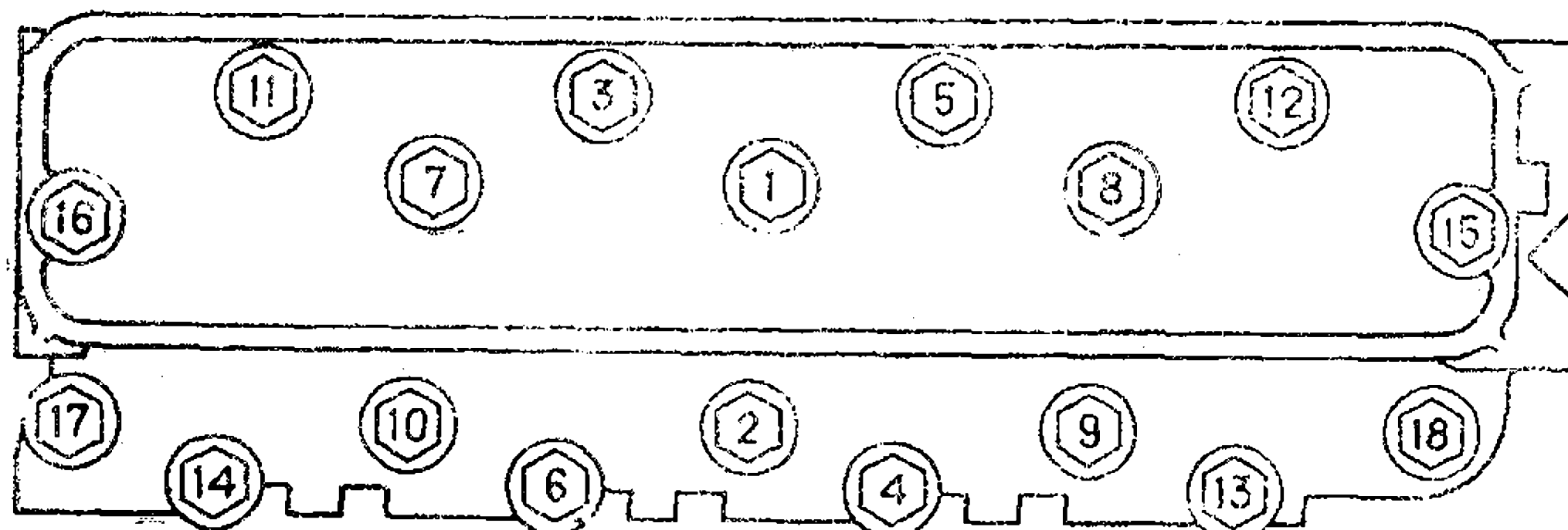
Рис. 7. Порядок затяжки гаек головки цилиндров
