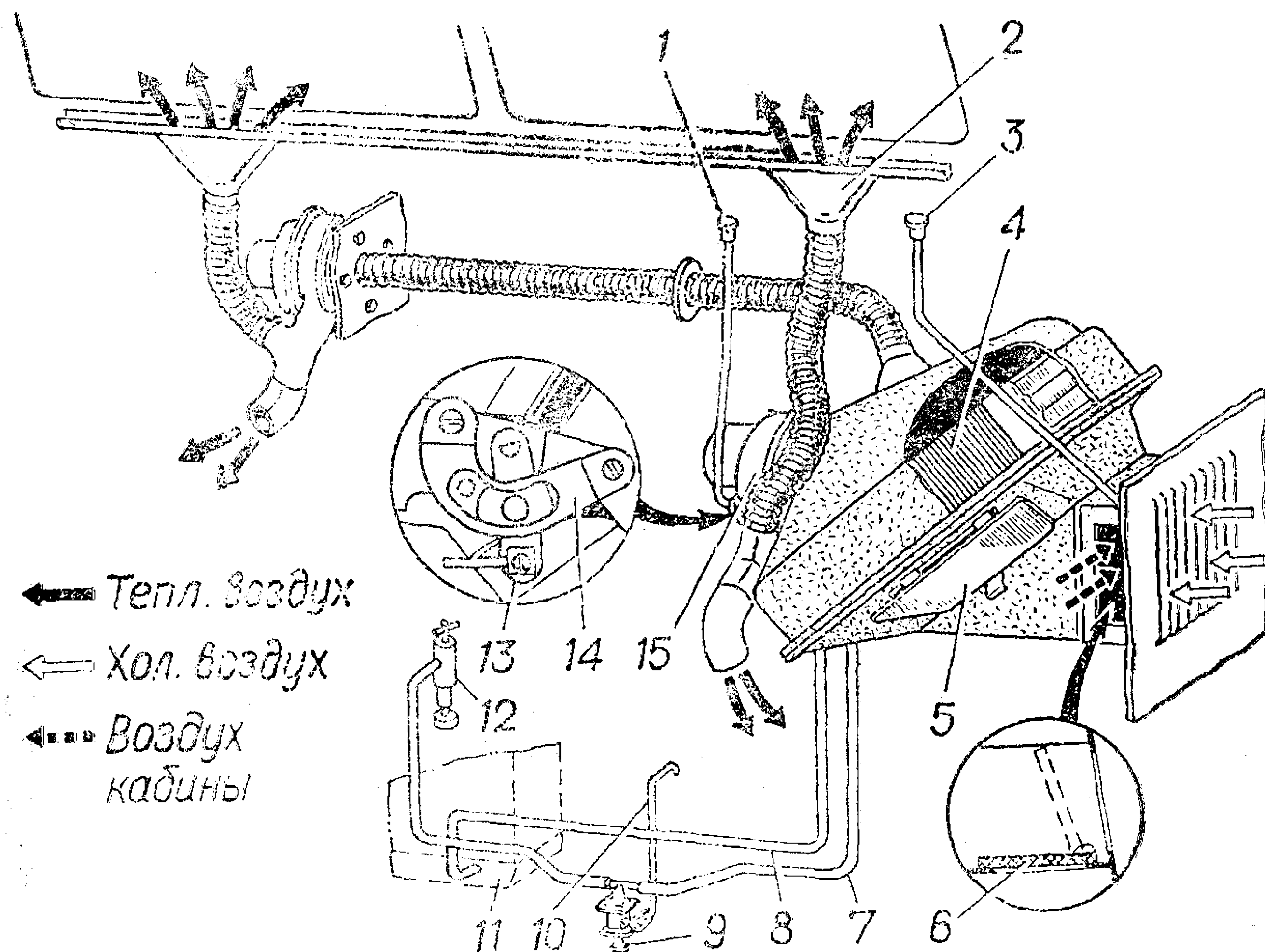
Рис. 76. Отопитель кабины:
