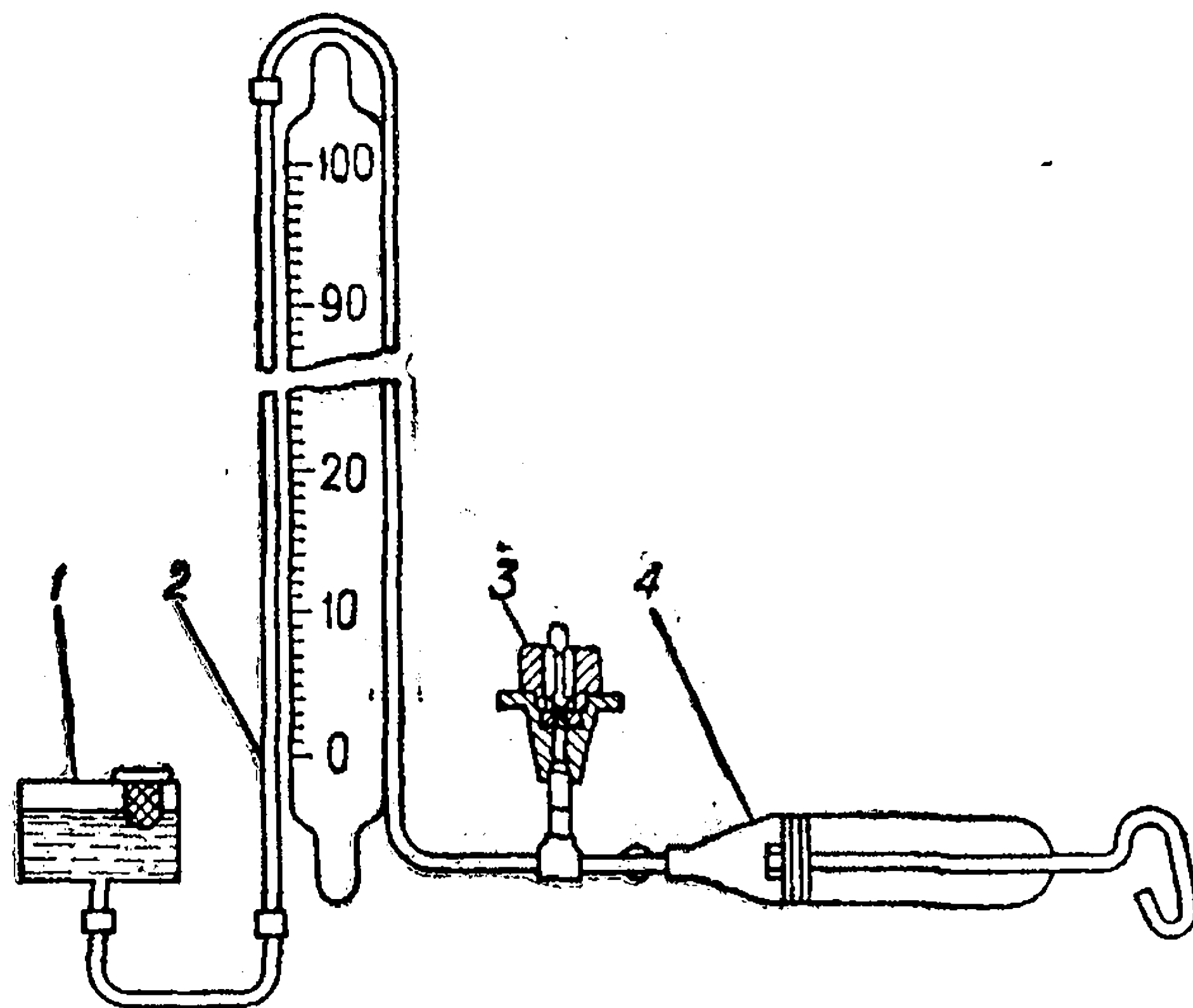
Рис. 84. Схема проверки герметичности топливного клапана:
