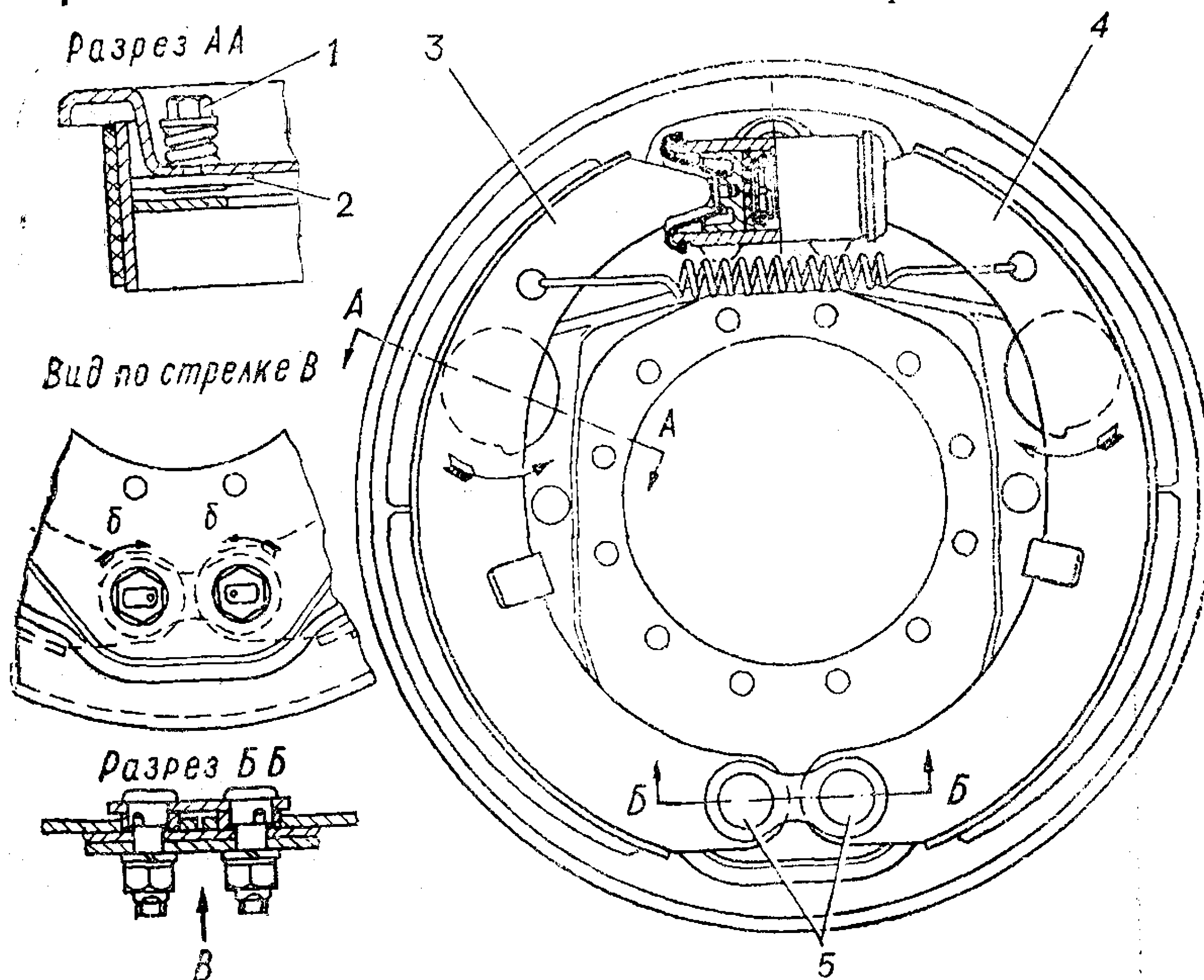
Рис. 94. Рабочий тормоз задних колес:
