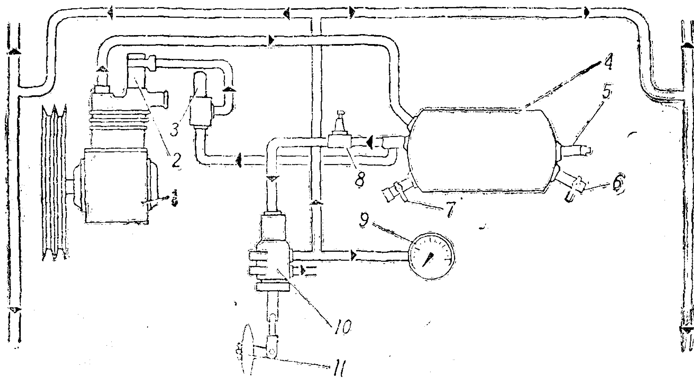
Рис. 38. Схема системы регулирования давления в шинах:
