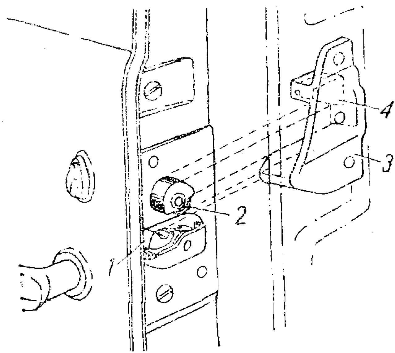
Рис. 73. Схема фиксации двери:
