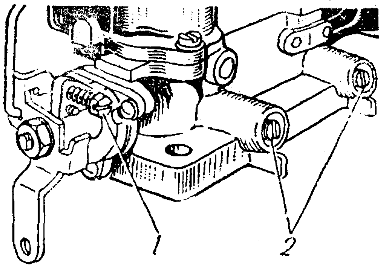
Рис. 87. Винты регулировки холостого хода:
