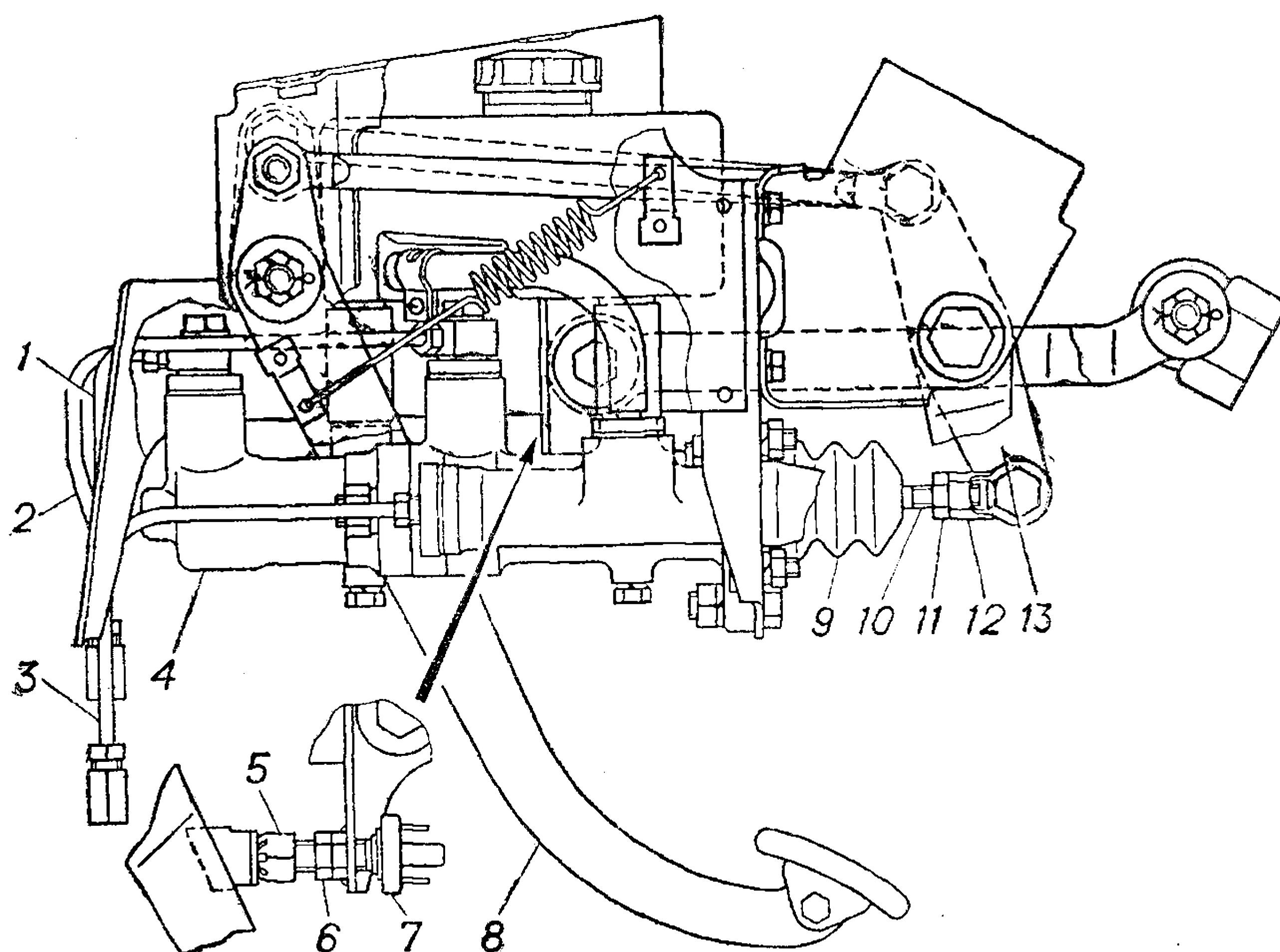
Рис. 97. Главный цилиндр тормоза и его привод:
