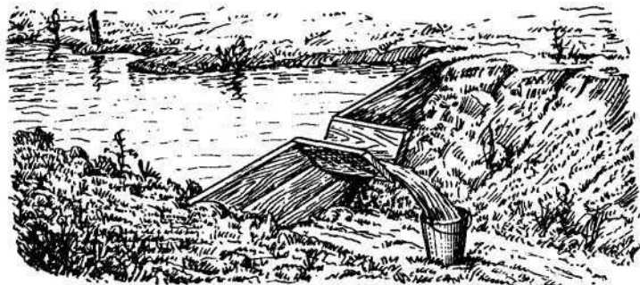
Измерение расхода воды при помощи перемычки с желобом
